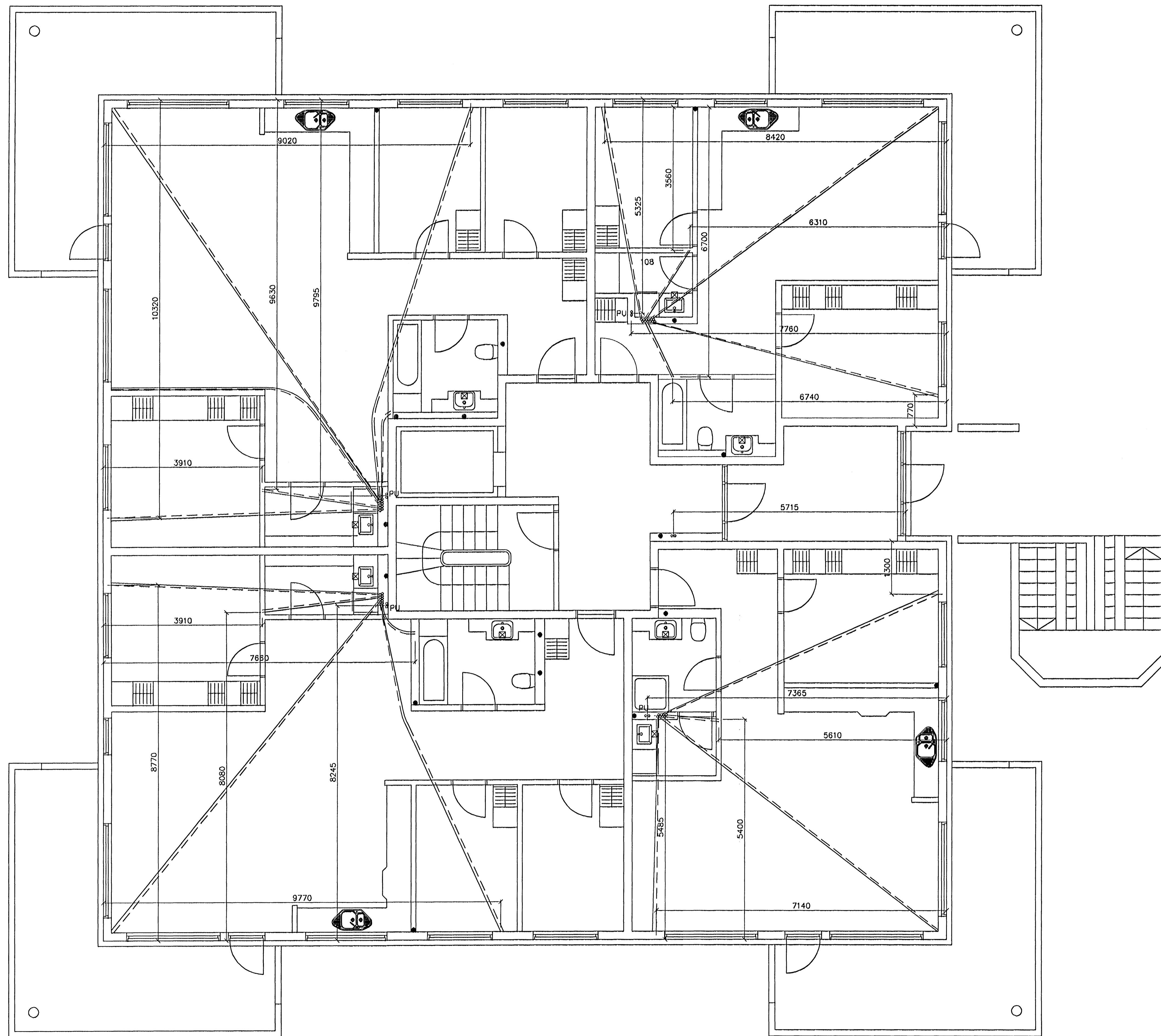
GRUNNMYND 1 HÆÐAR 1:50
