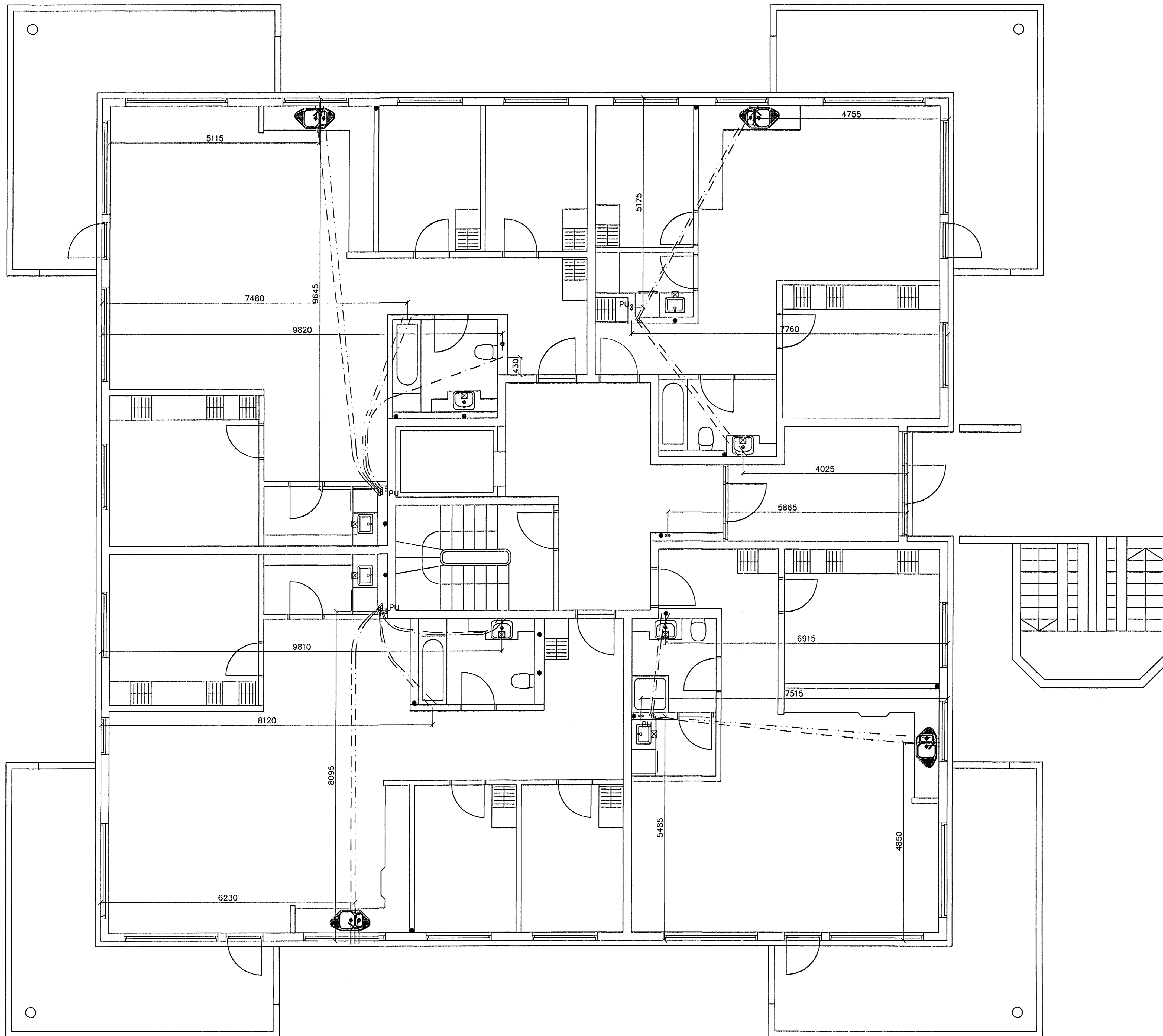
GRUNNMYND 1 HÆÐAR 1:50
