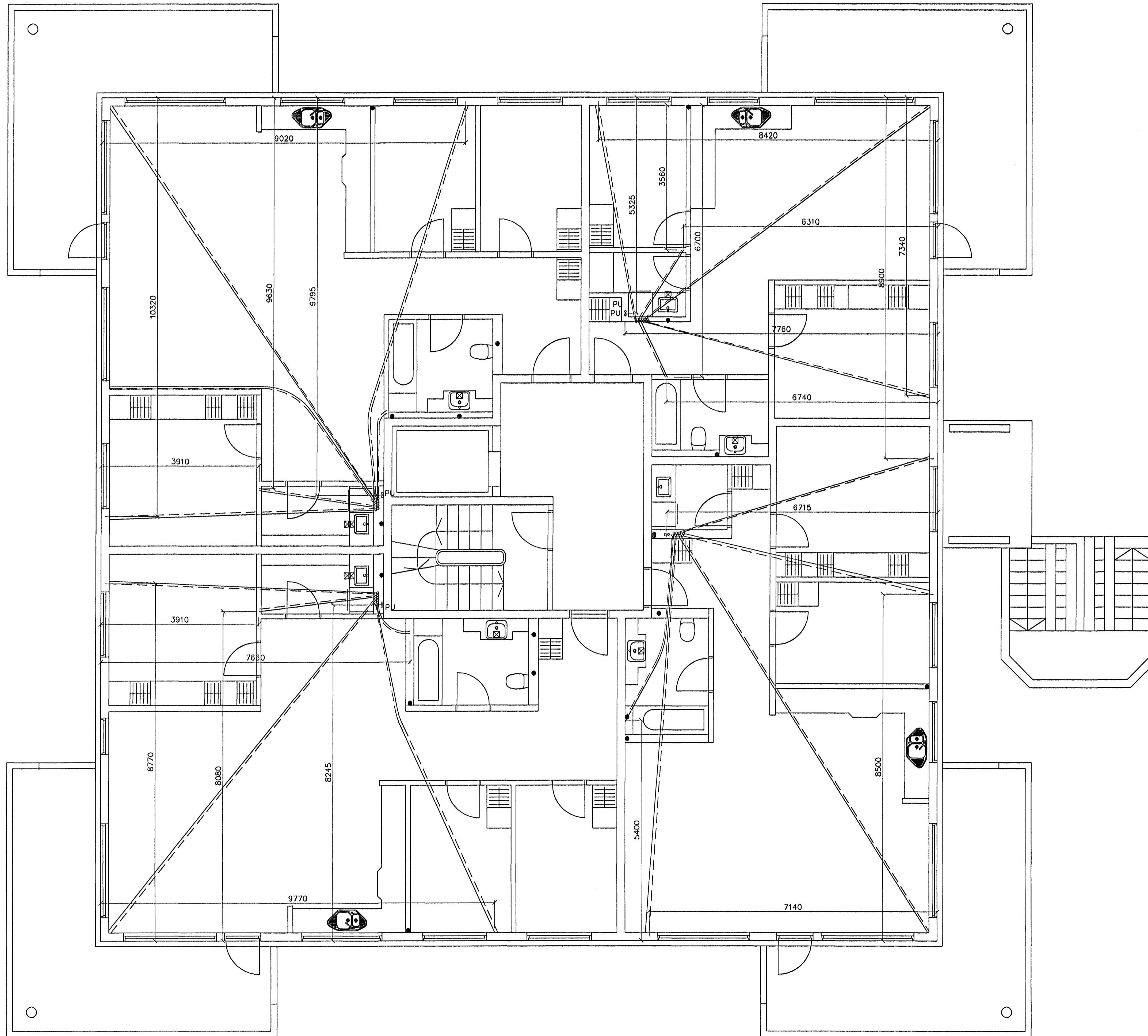
GRUNNMYND 6 HÆÐAR 1:50
