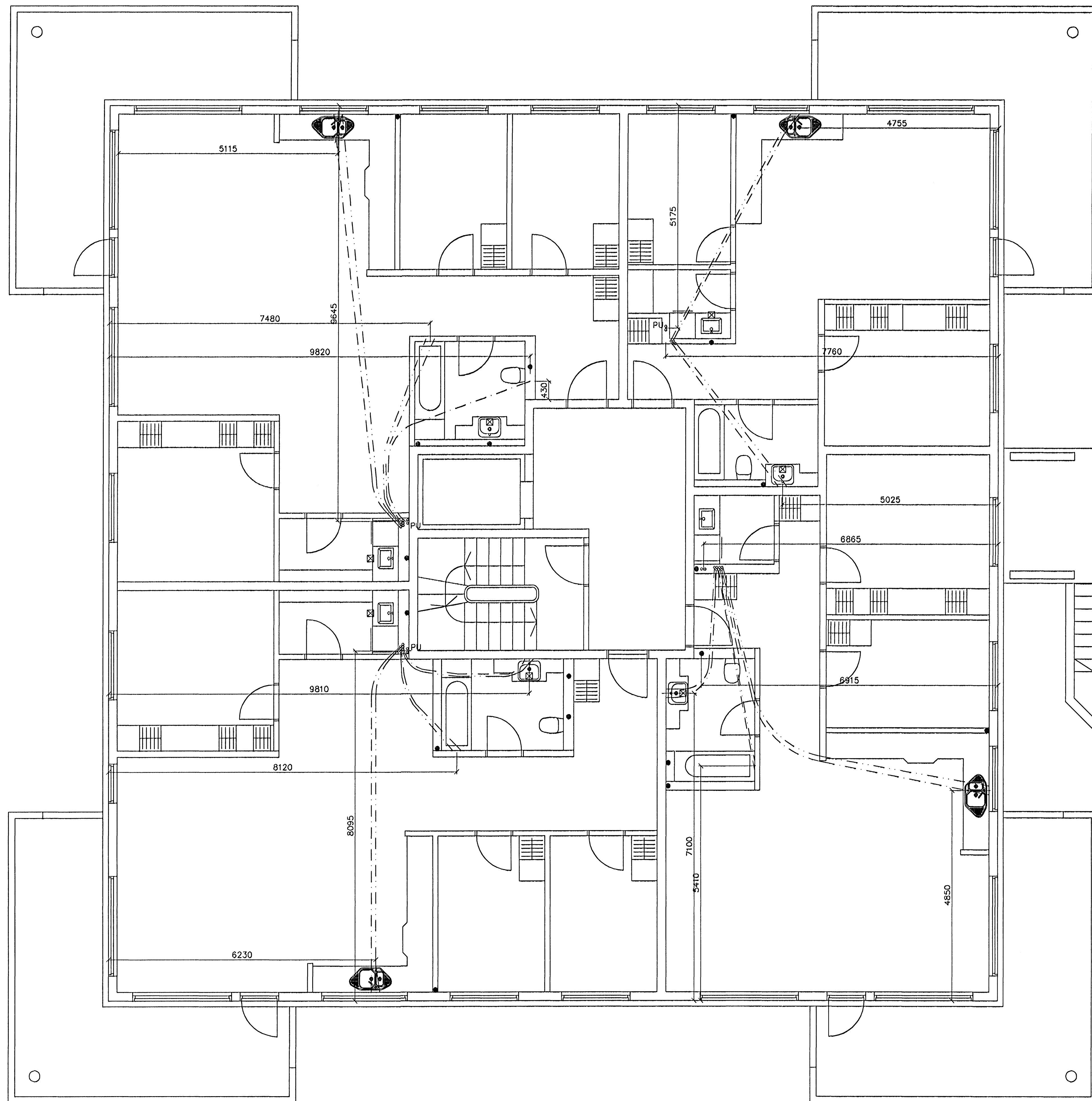
GRUNNMYND 6 HÆÐAR 1:50
