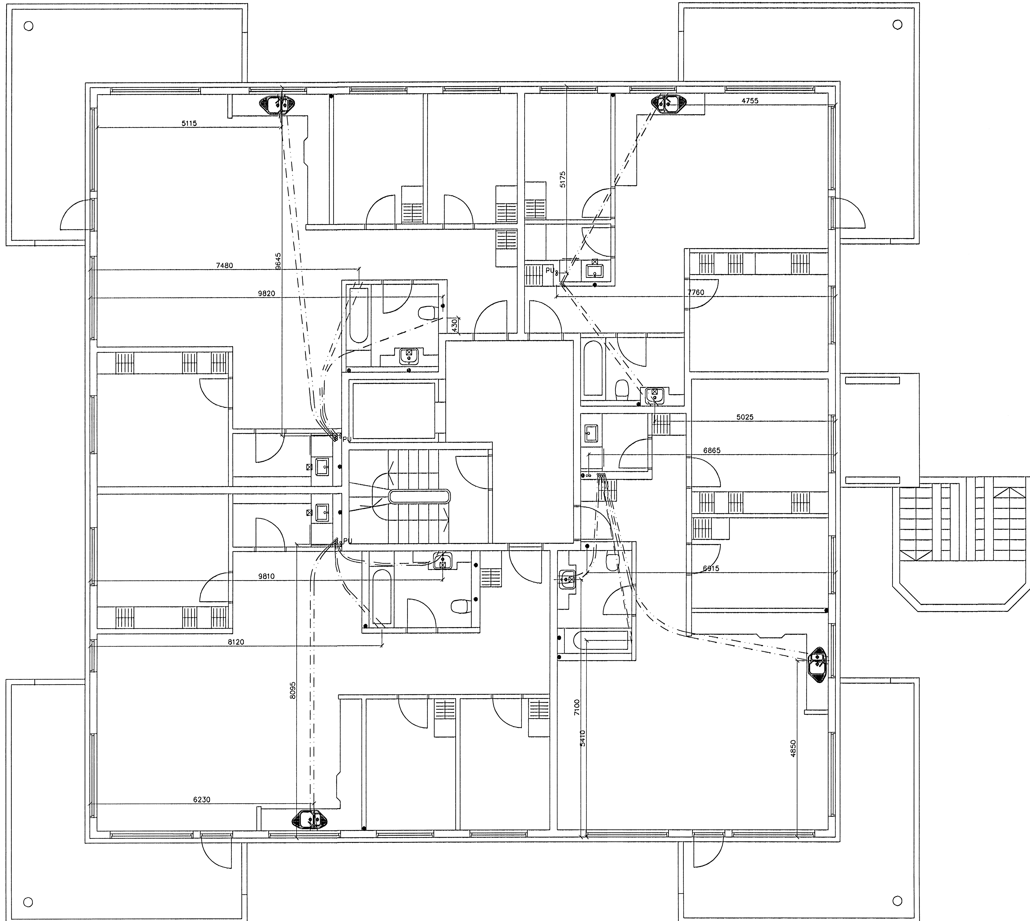
GRUNNMYND 5 HÆÐAR 1:50
