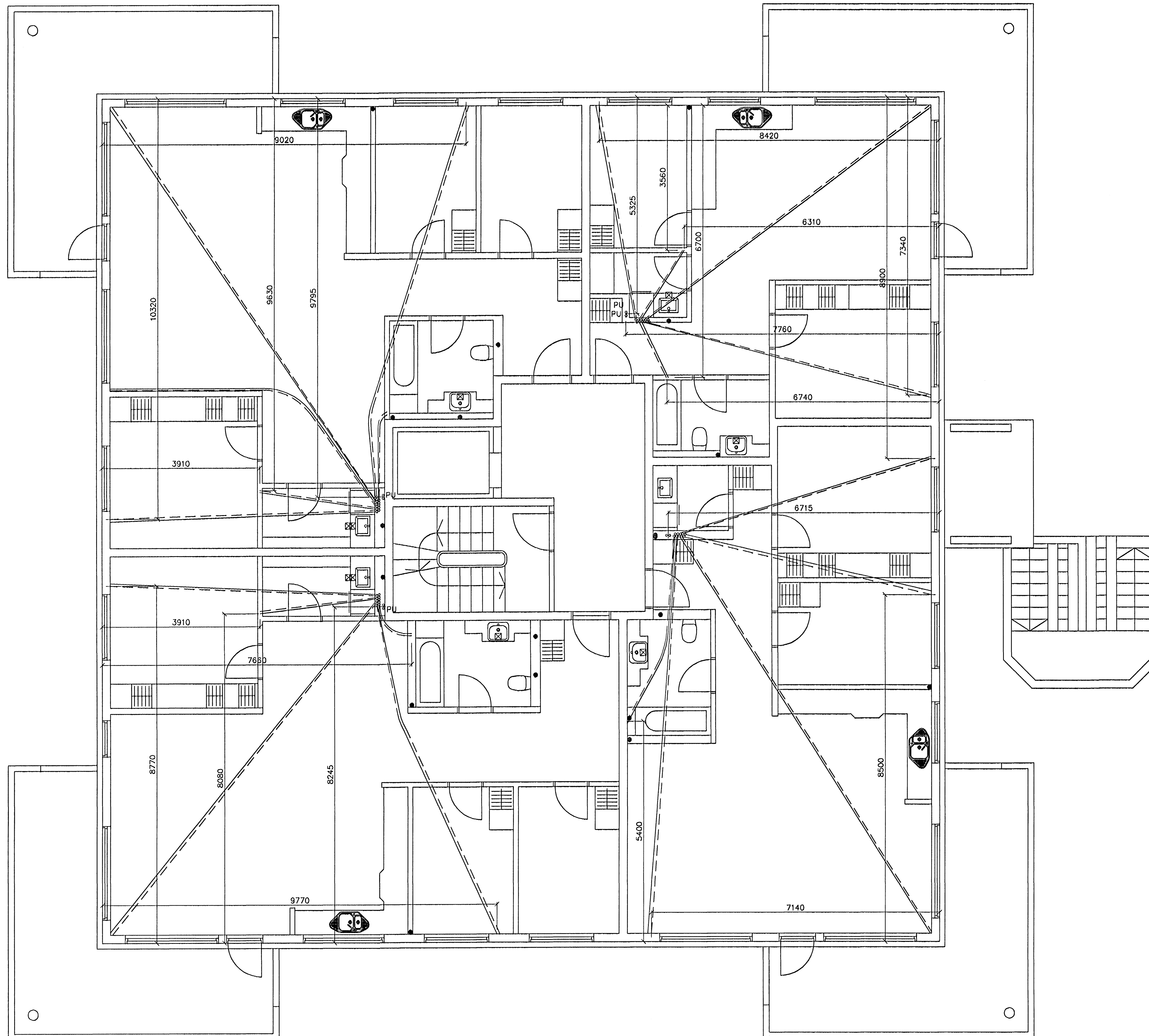
GRUNNMYND 4 HÆÐAR 1:50
