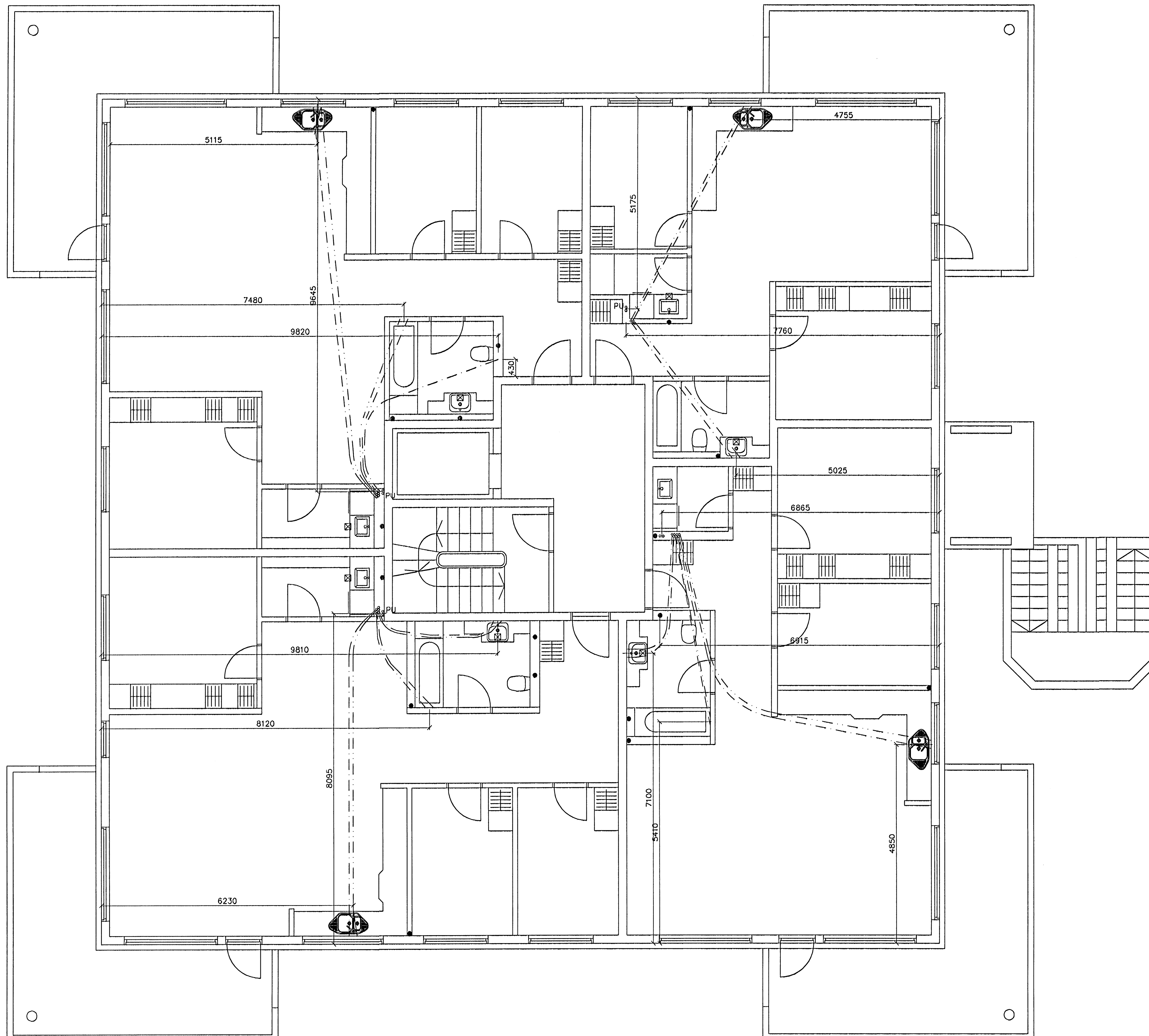
GRUNNMYND 4 HÆÐAR 1:50
