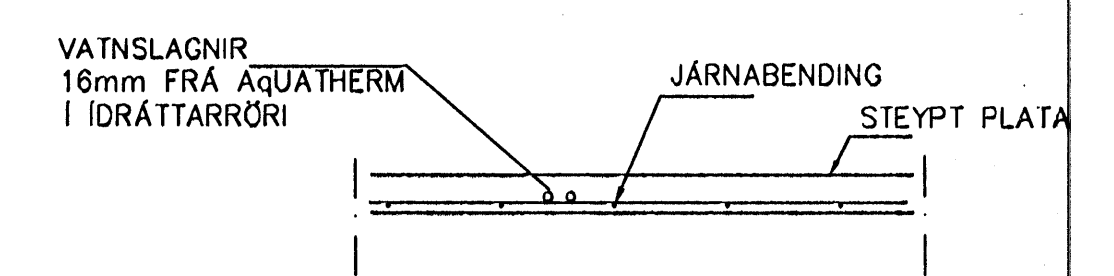
LAGNIR, SNIÐ, 1:20
