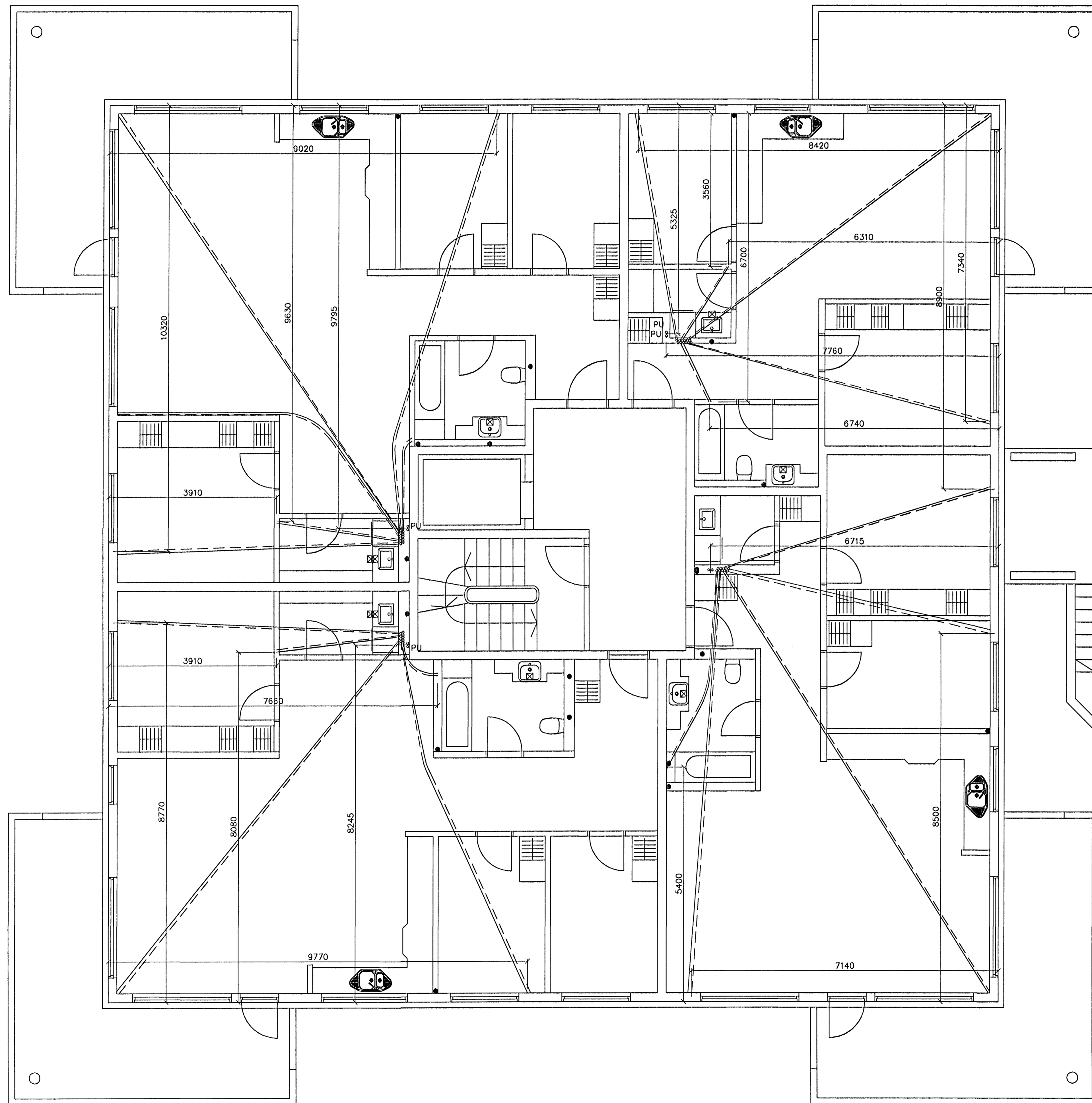
GRUNNMYND 2 HÆÐAR 1:50
