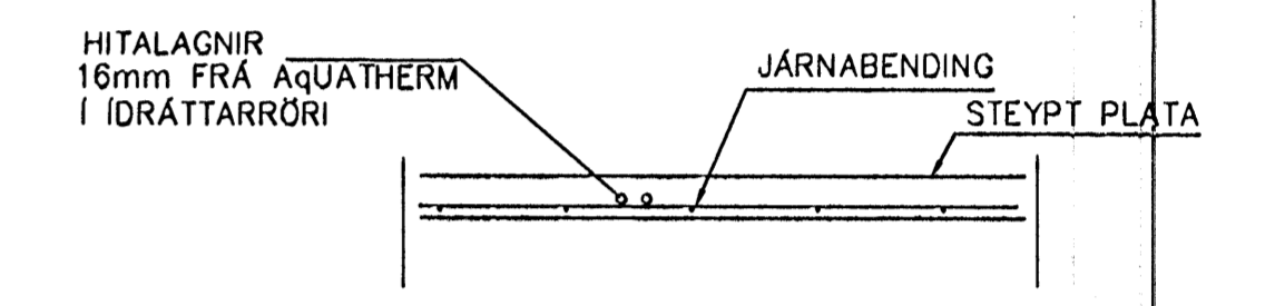
LAGNIR, SNIÐ, 1:20
