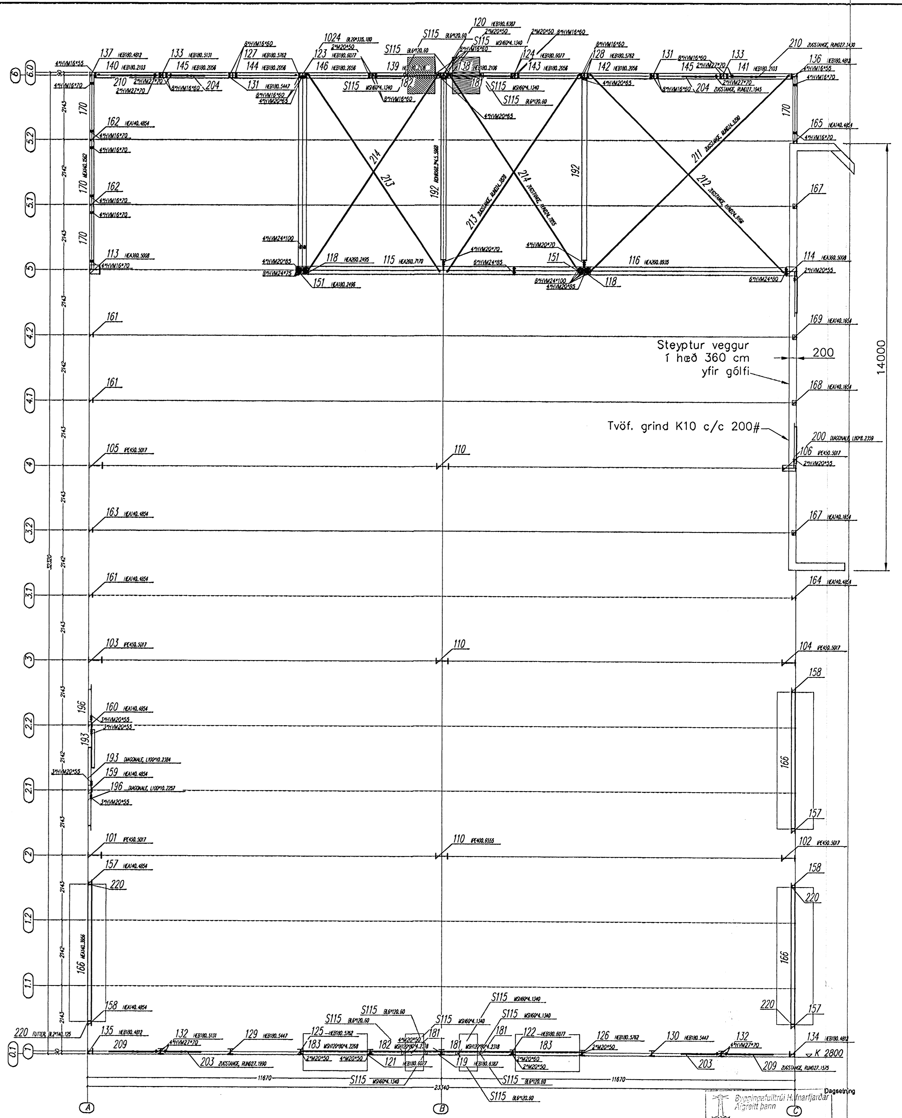
Grunnmynd kóti +2800
