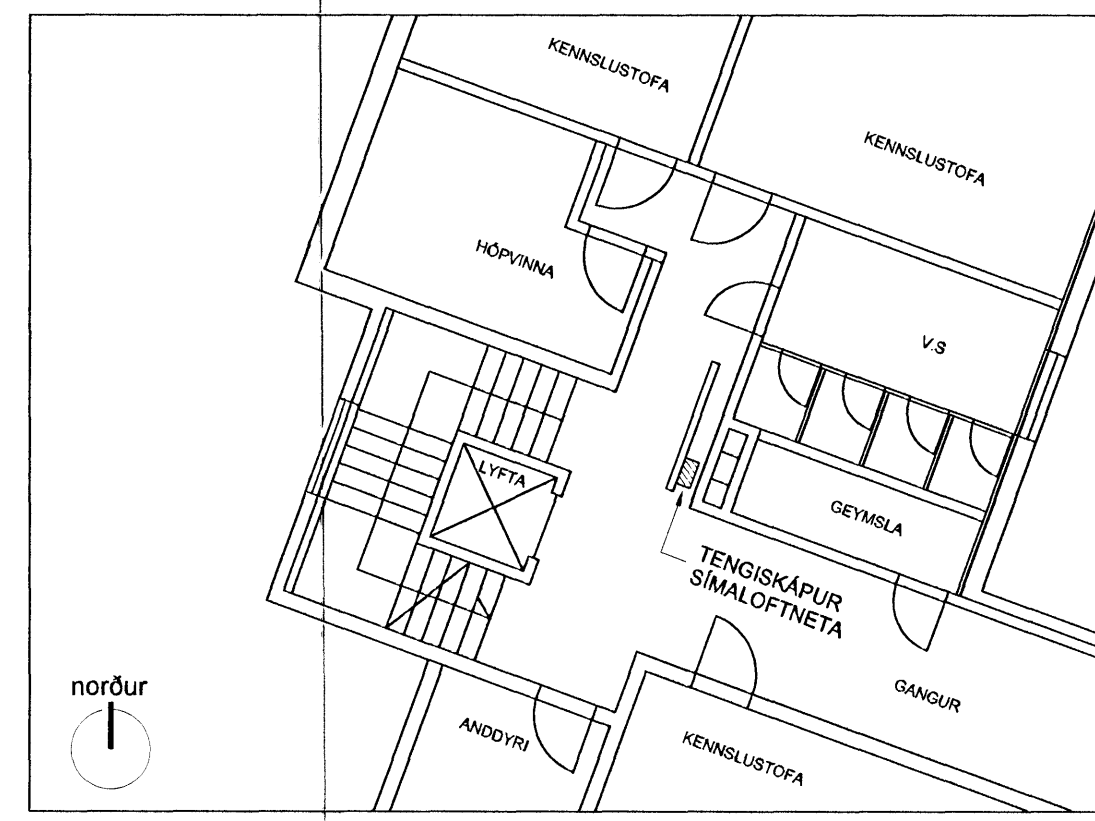
GRUNNMYND mkv 1:100
