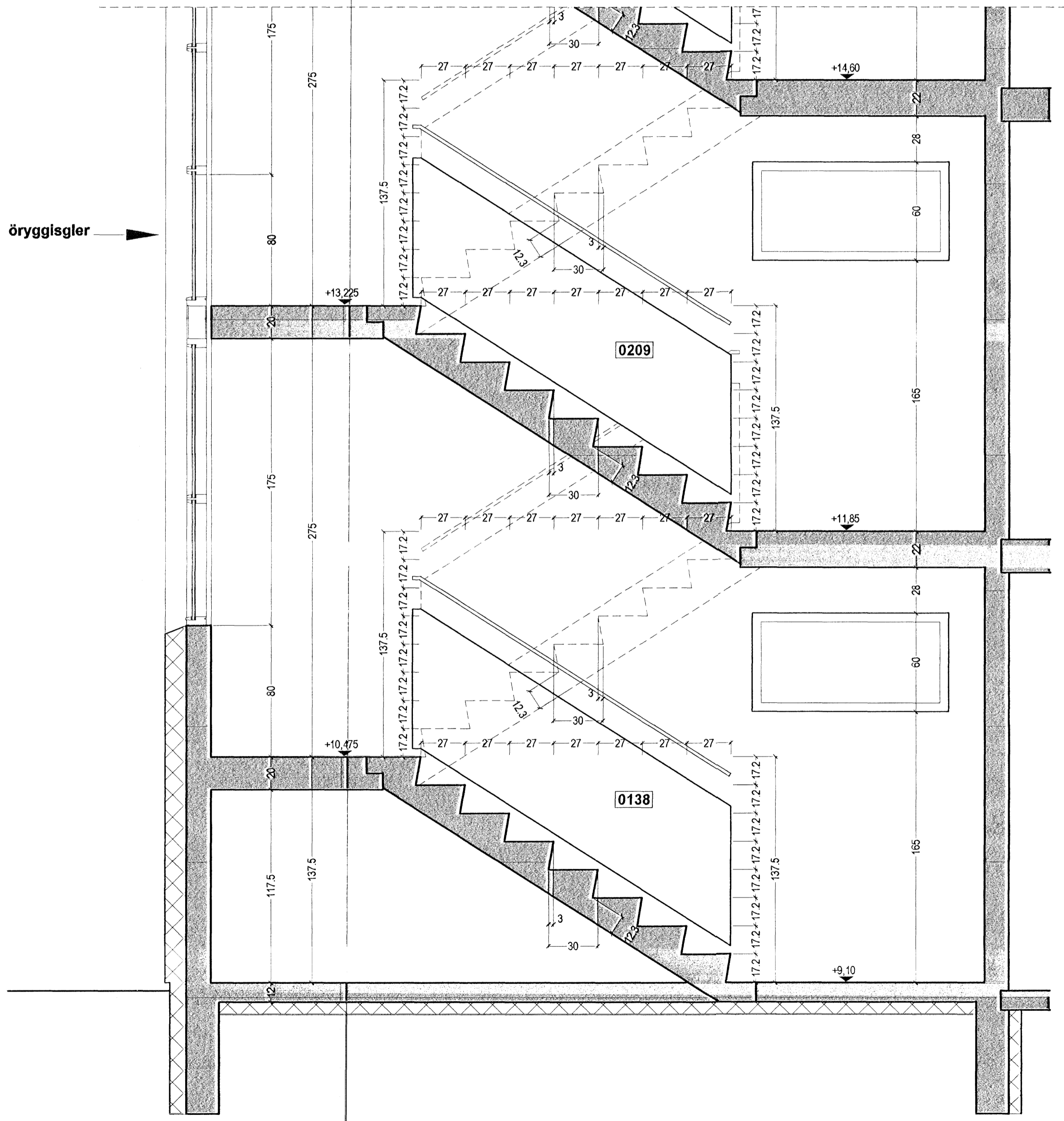
Snið A-A
