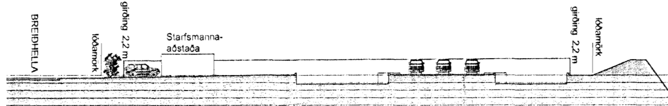
SKURÐUR A-A M 1:500
