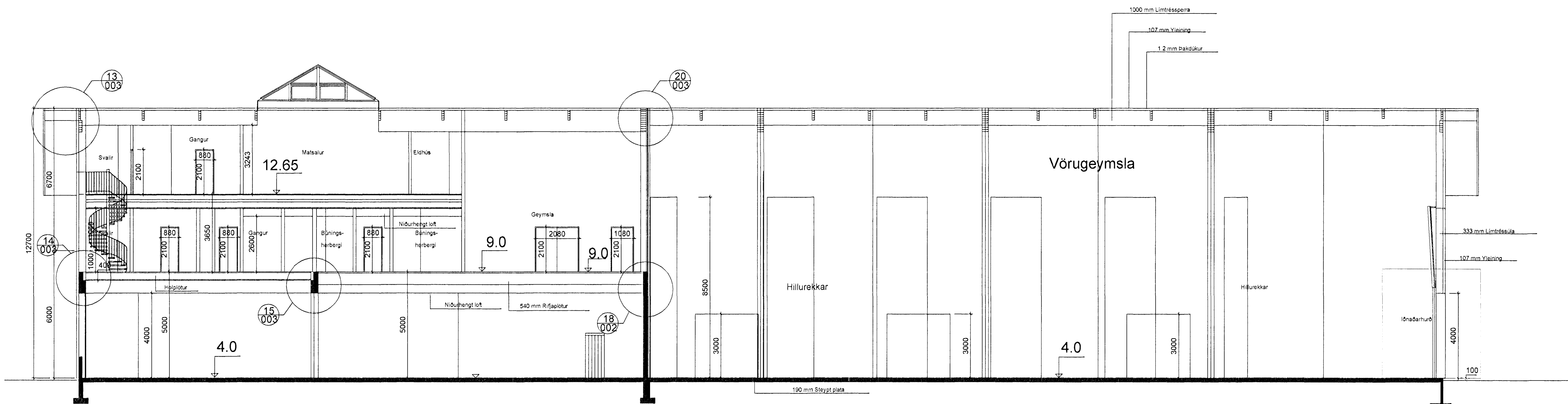
Skurður D-D
