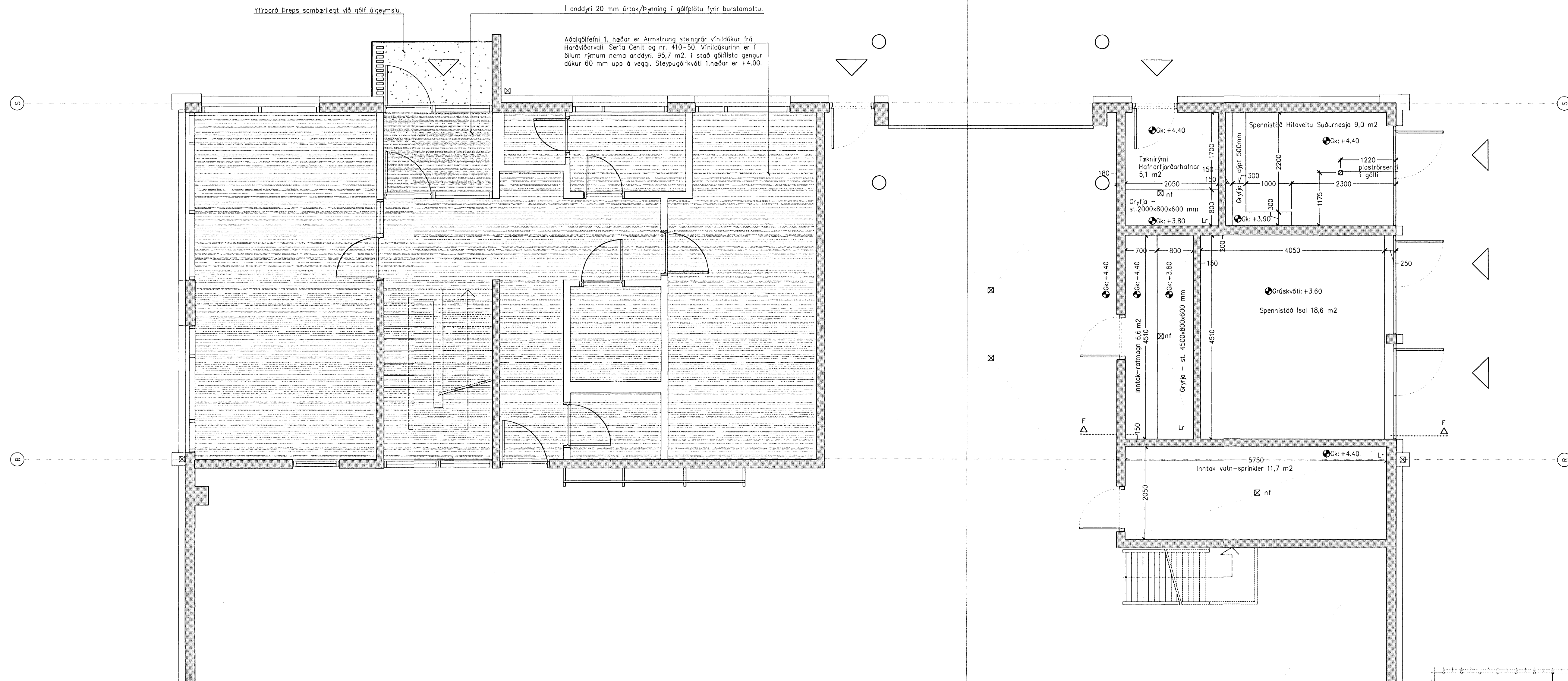
Gólfefnayfirlit 1.hæðar - mkv. 1: 50
