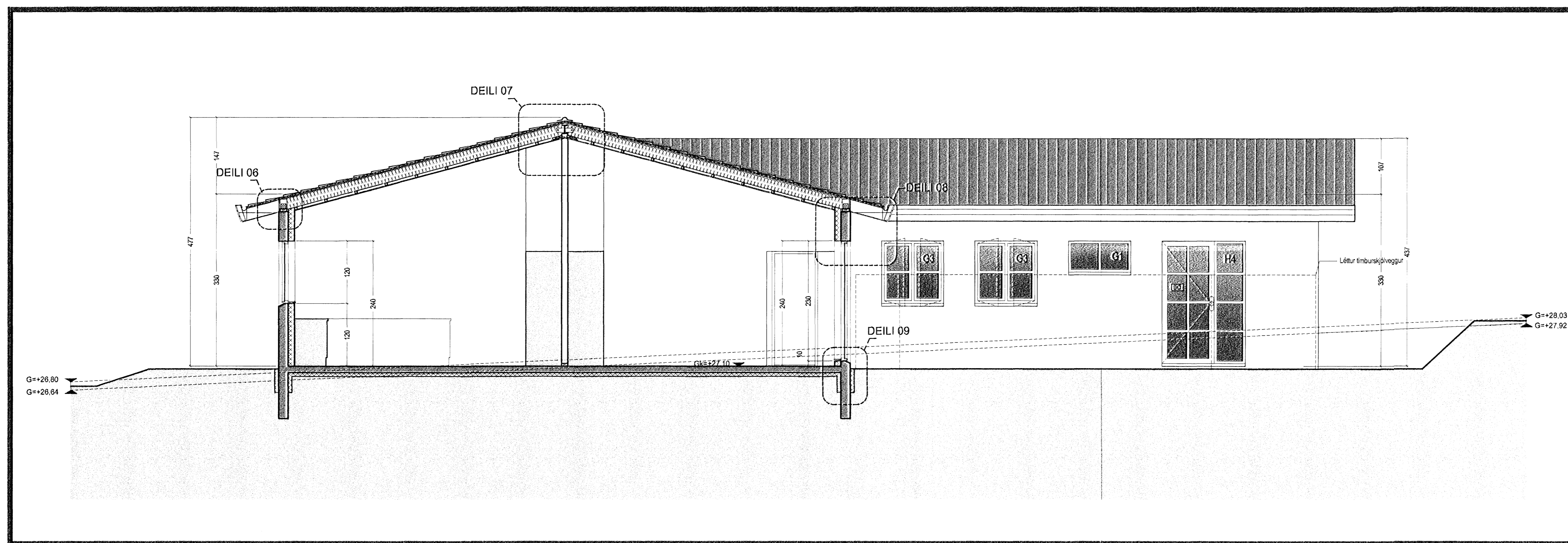
Snið 3 1:50
