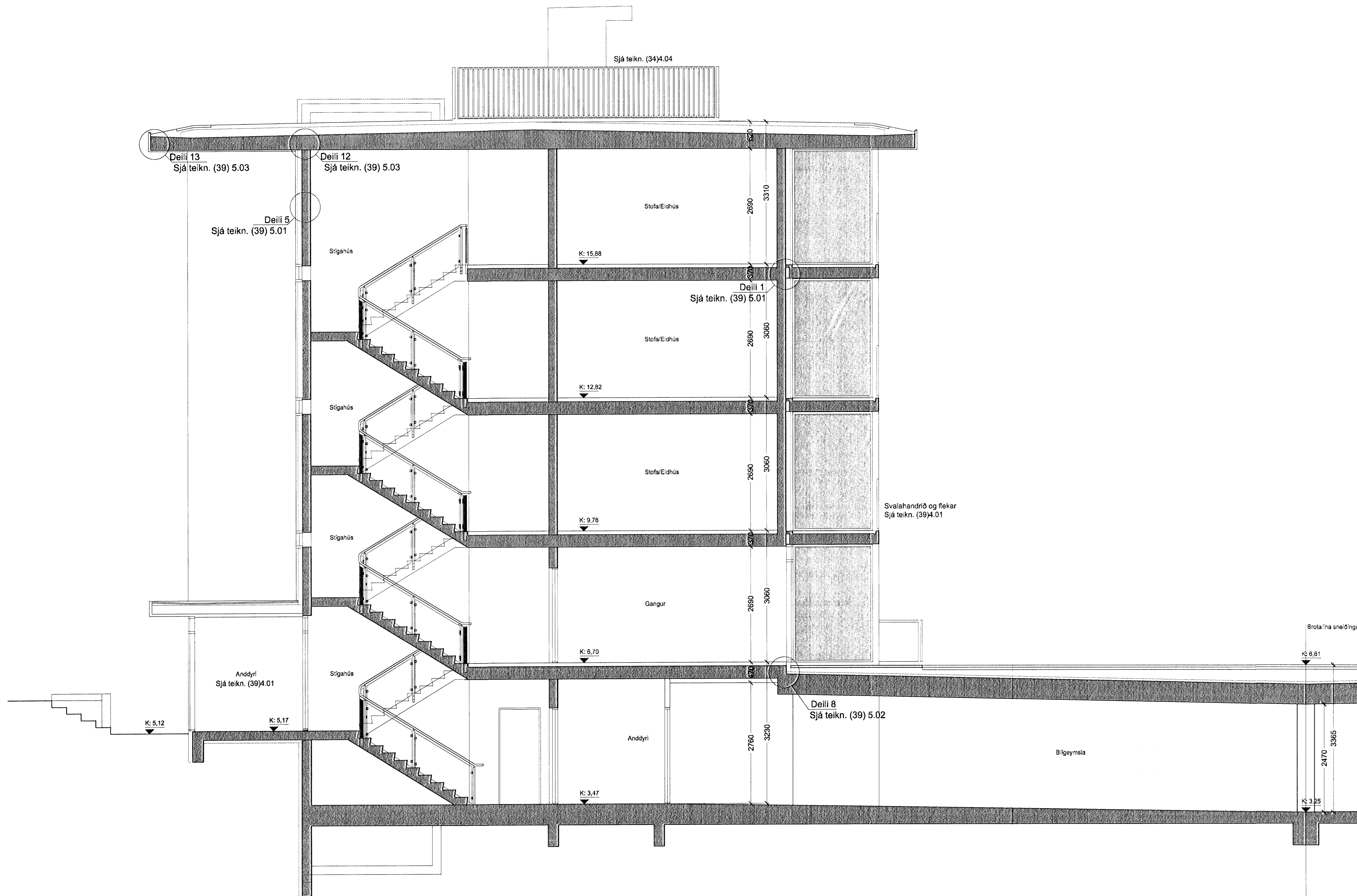
SNID A-A í mkv. 1:50
