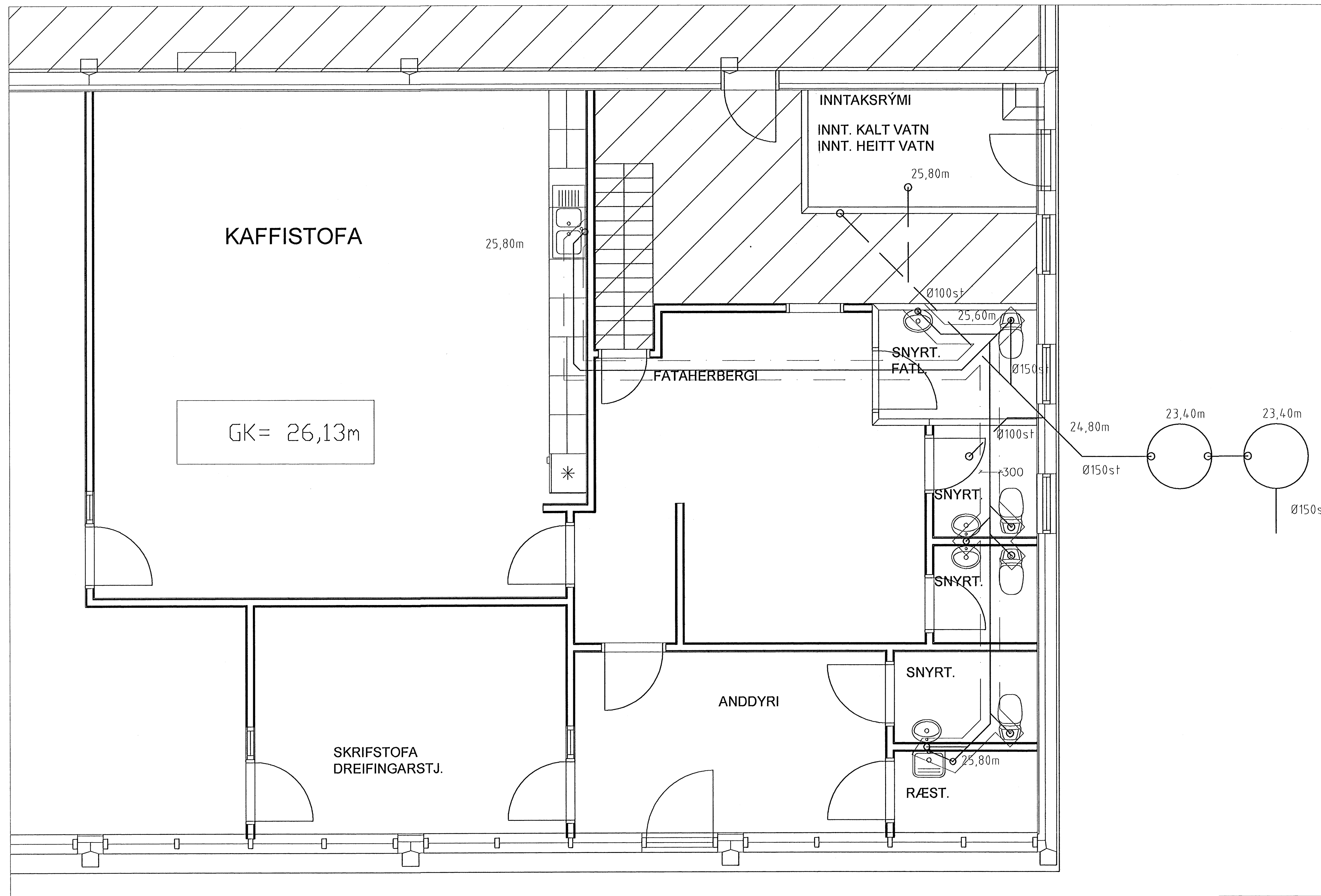
Grunnmynd 1:50
