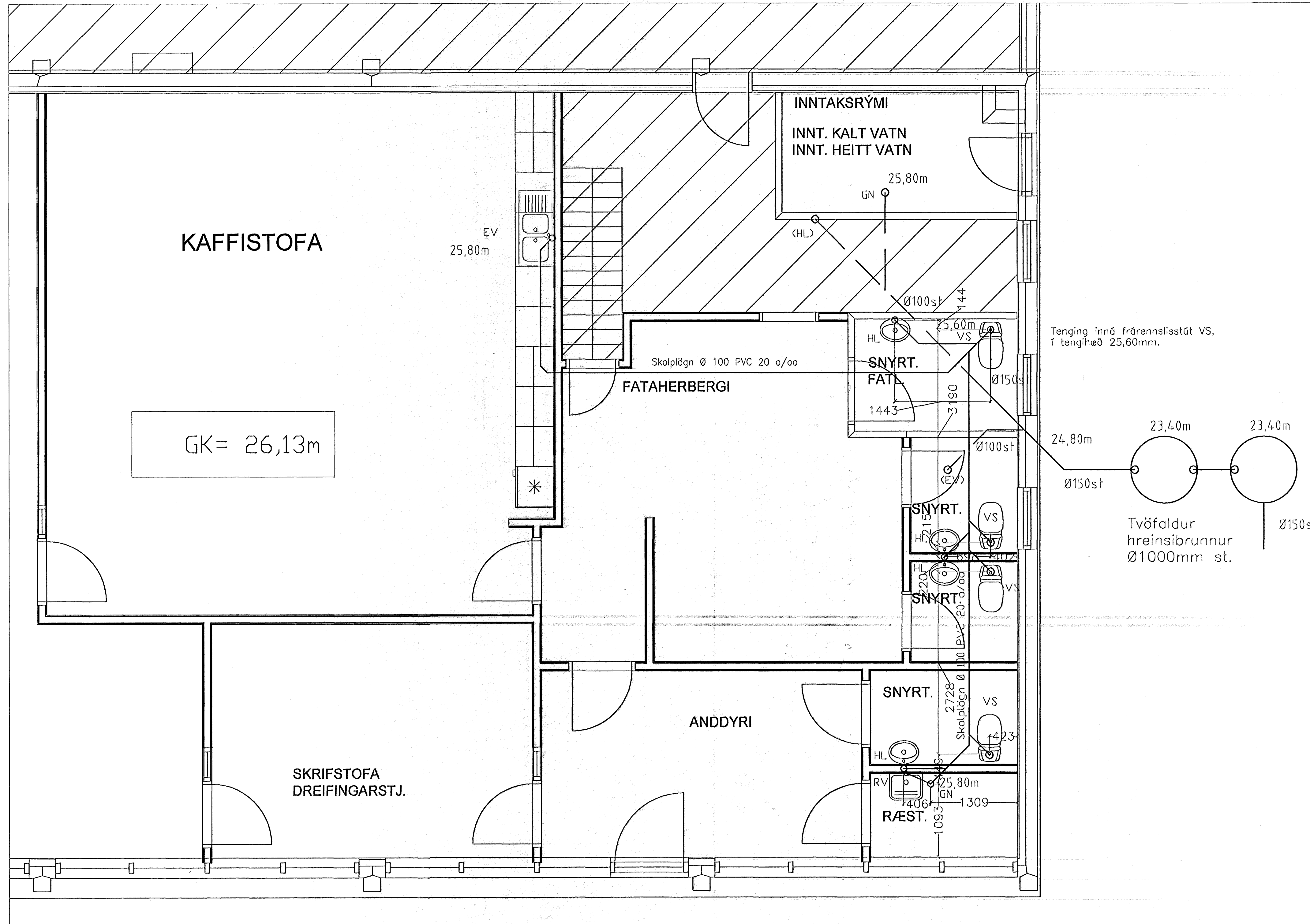
Grunnmynd 1:50
