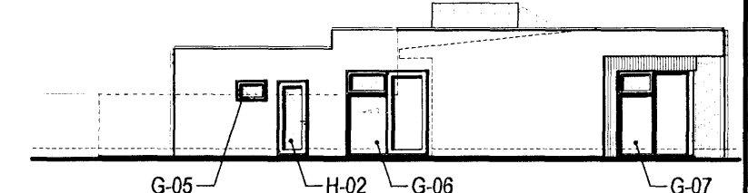
Suður M= 1:200
