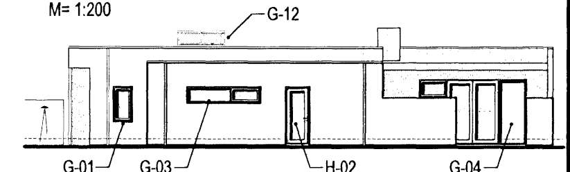
Vestur M= 1:200
