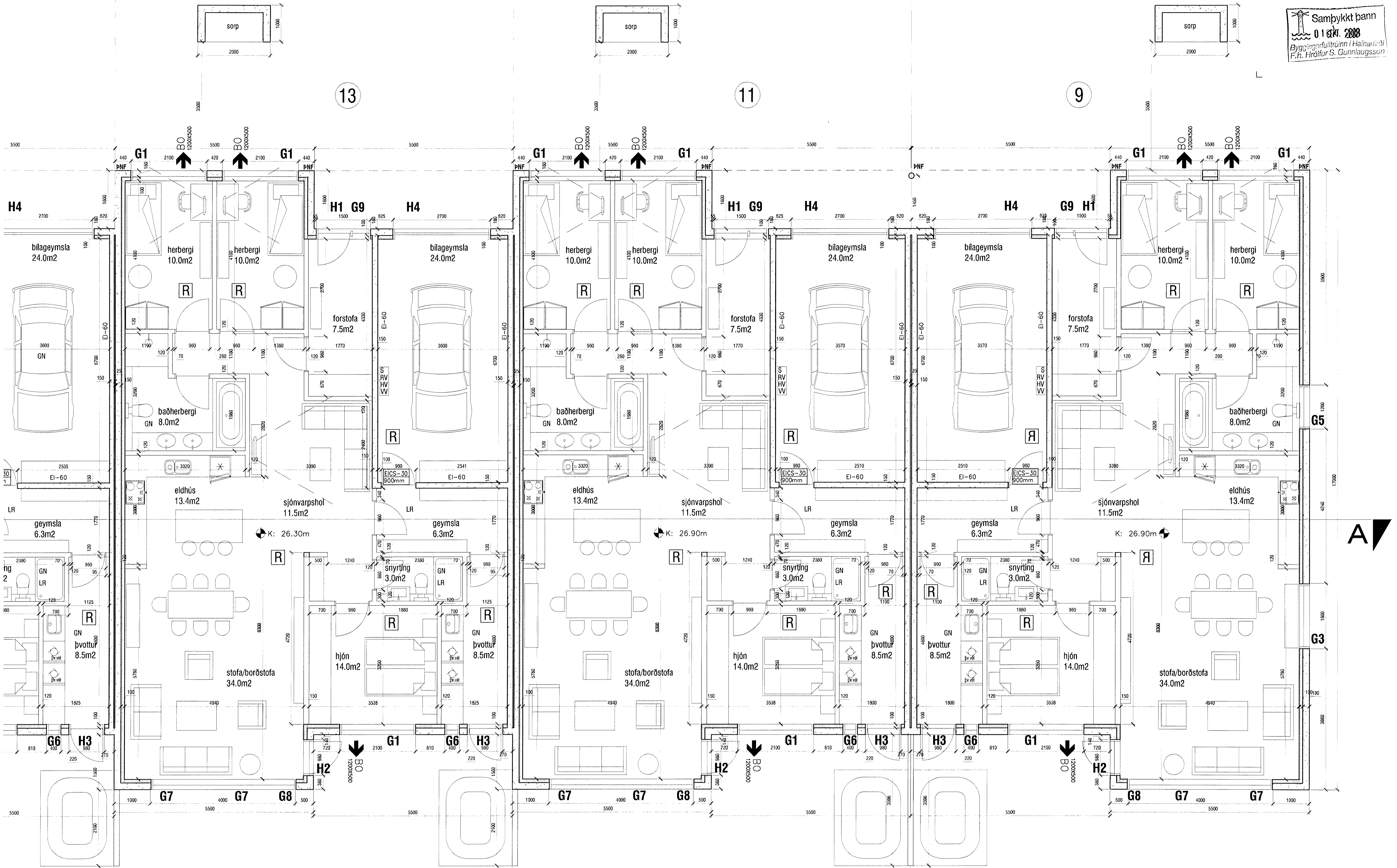
Grunnmynd - 13 mkv. 1:100
