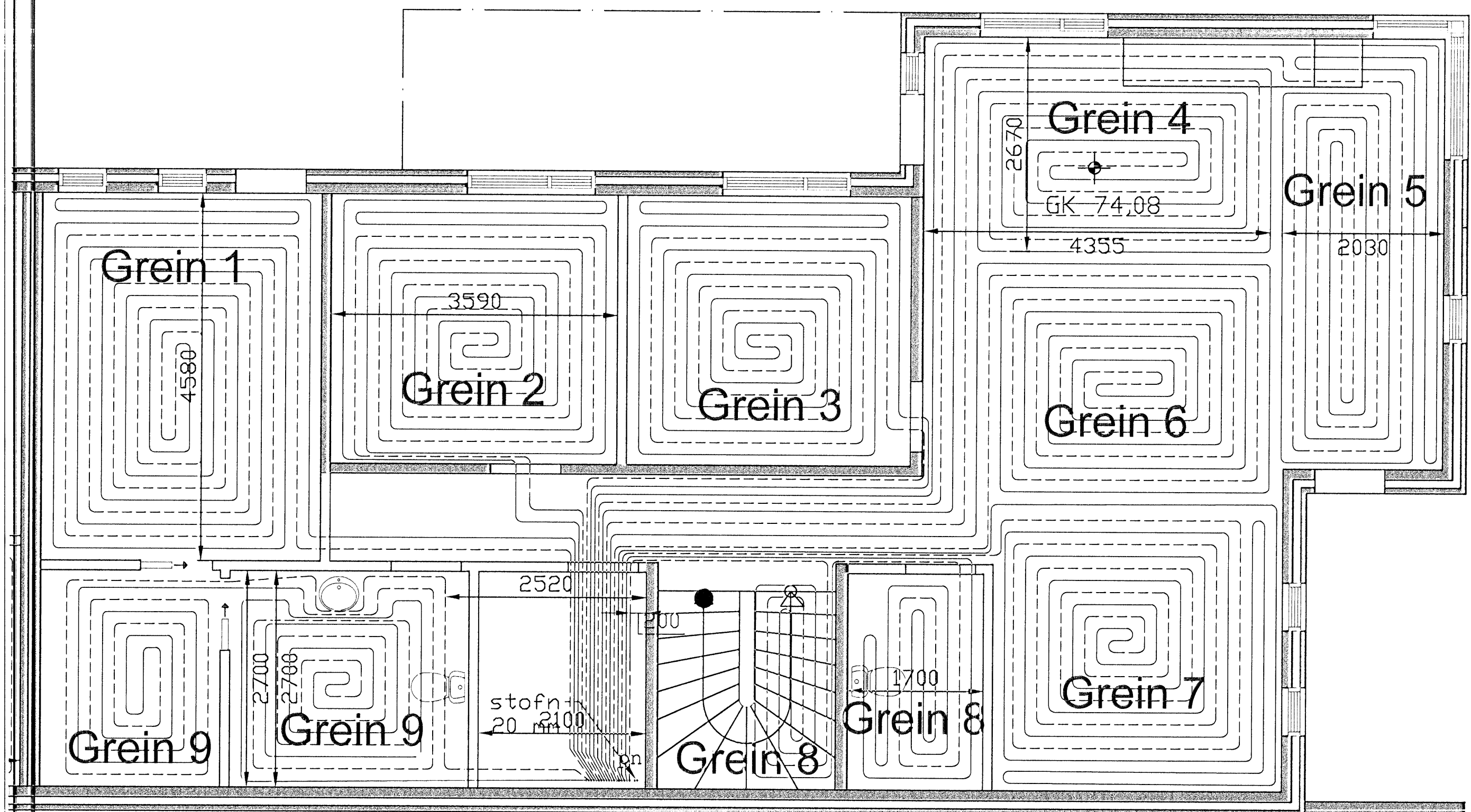
Grunnmynd 1. hæð Furuás 5 Kvarði 1:50
