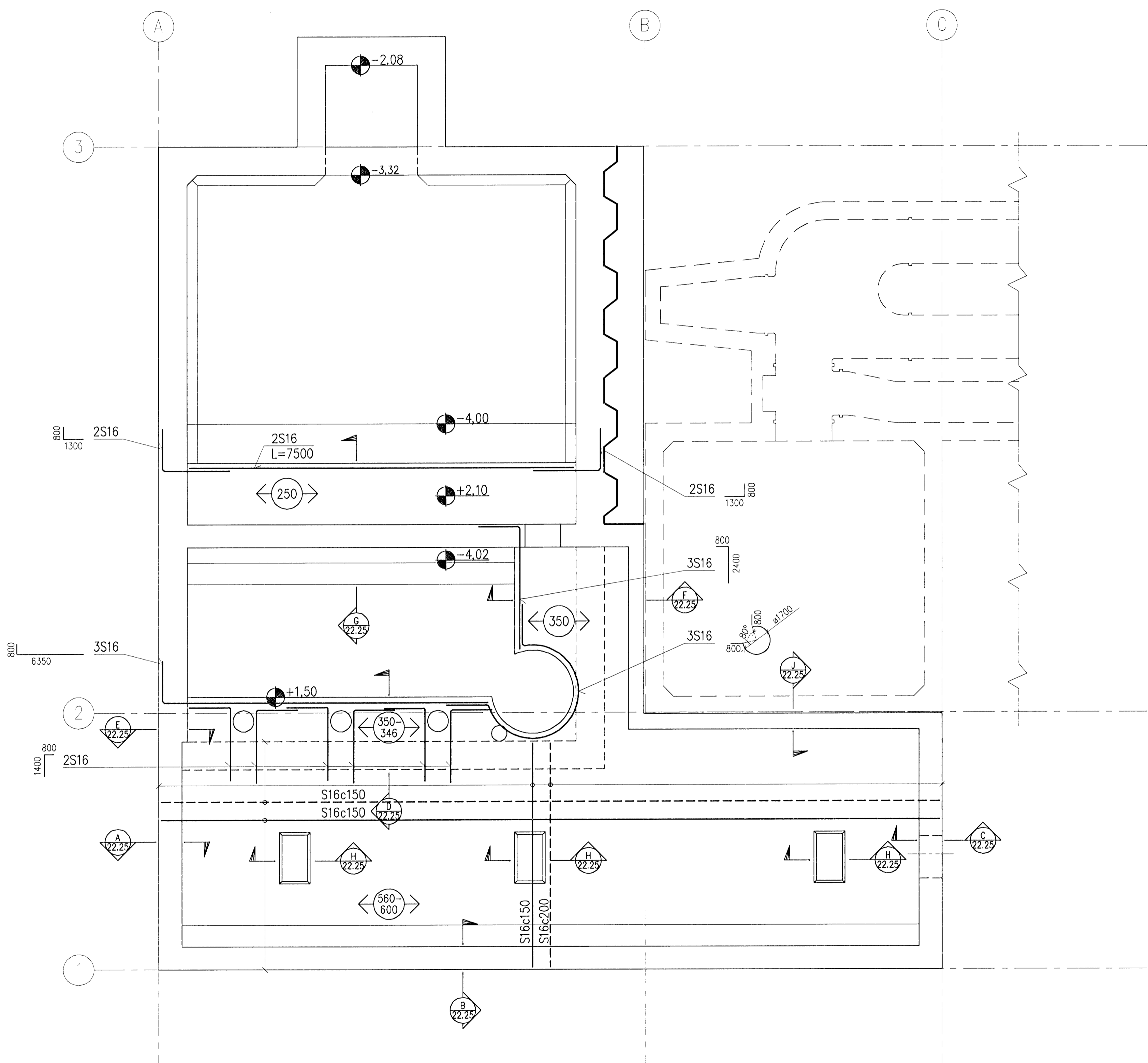
GRUNNMYND BOTNPLÖTU (K.+1.50)
