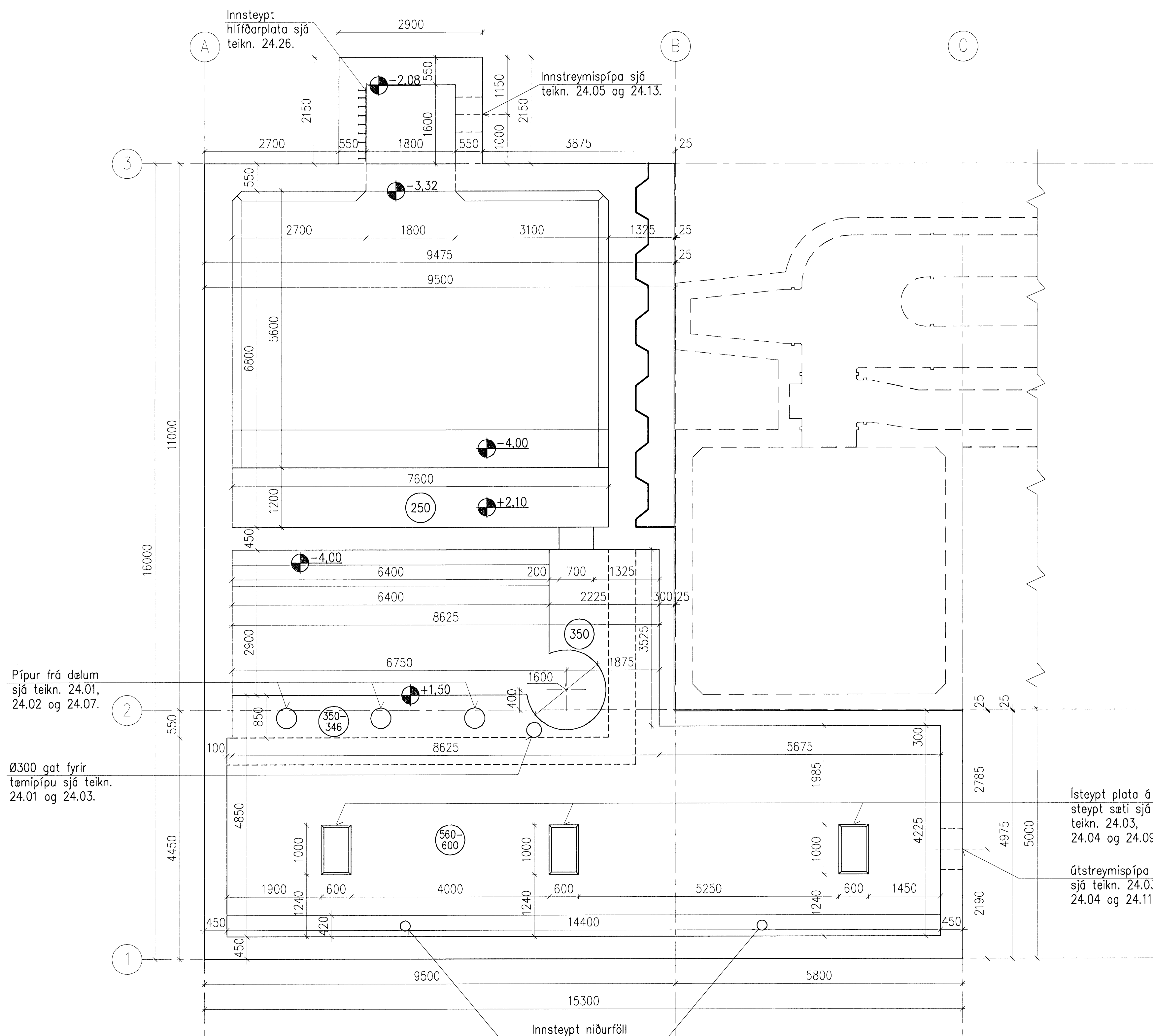
GRUNNMYND BOTNPLÖTU (K.+1.50)
