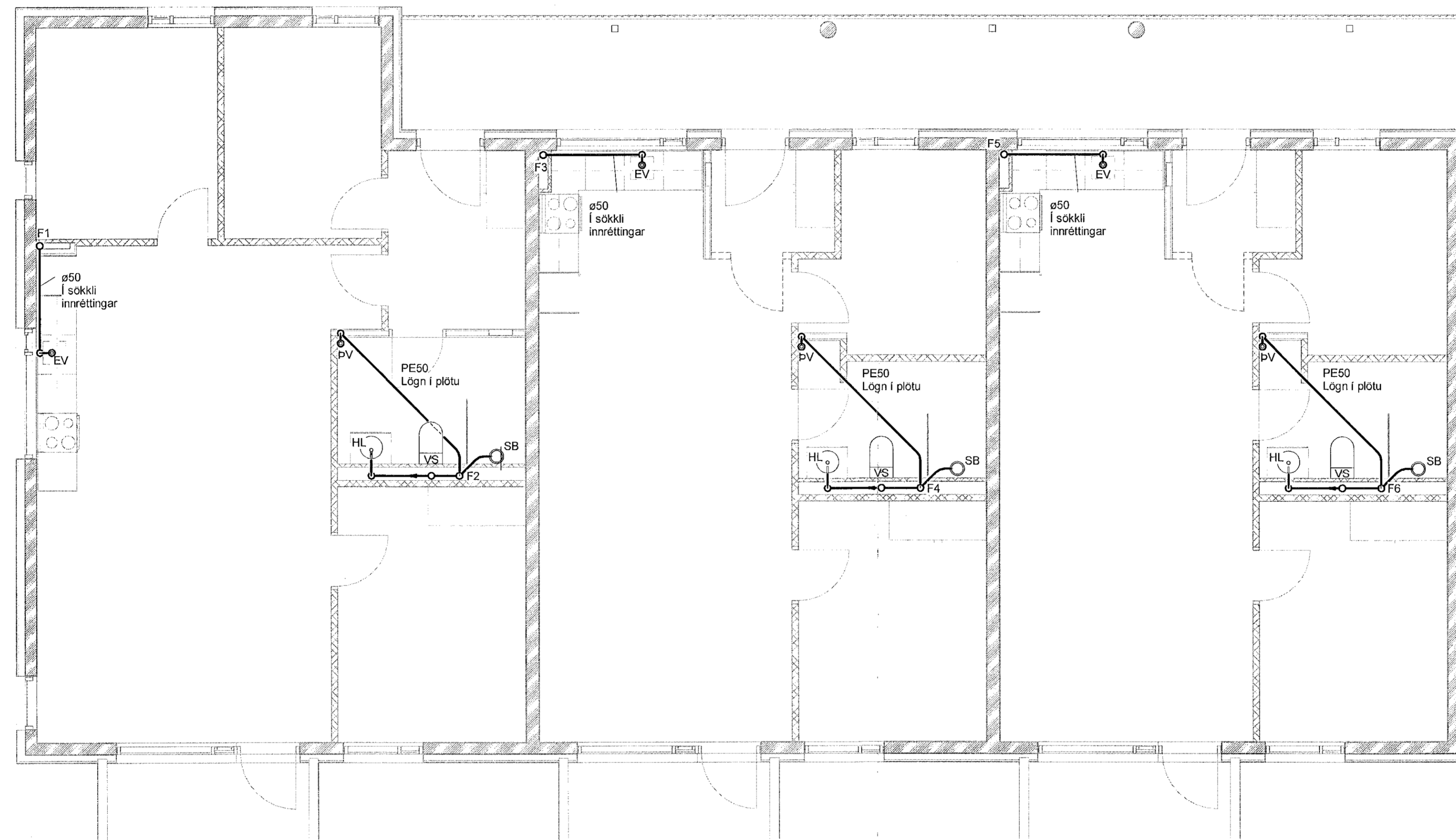
1 3. hæð - 1 1 : 50
