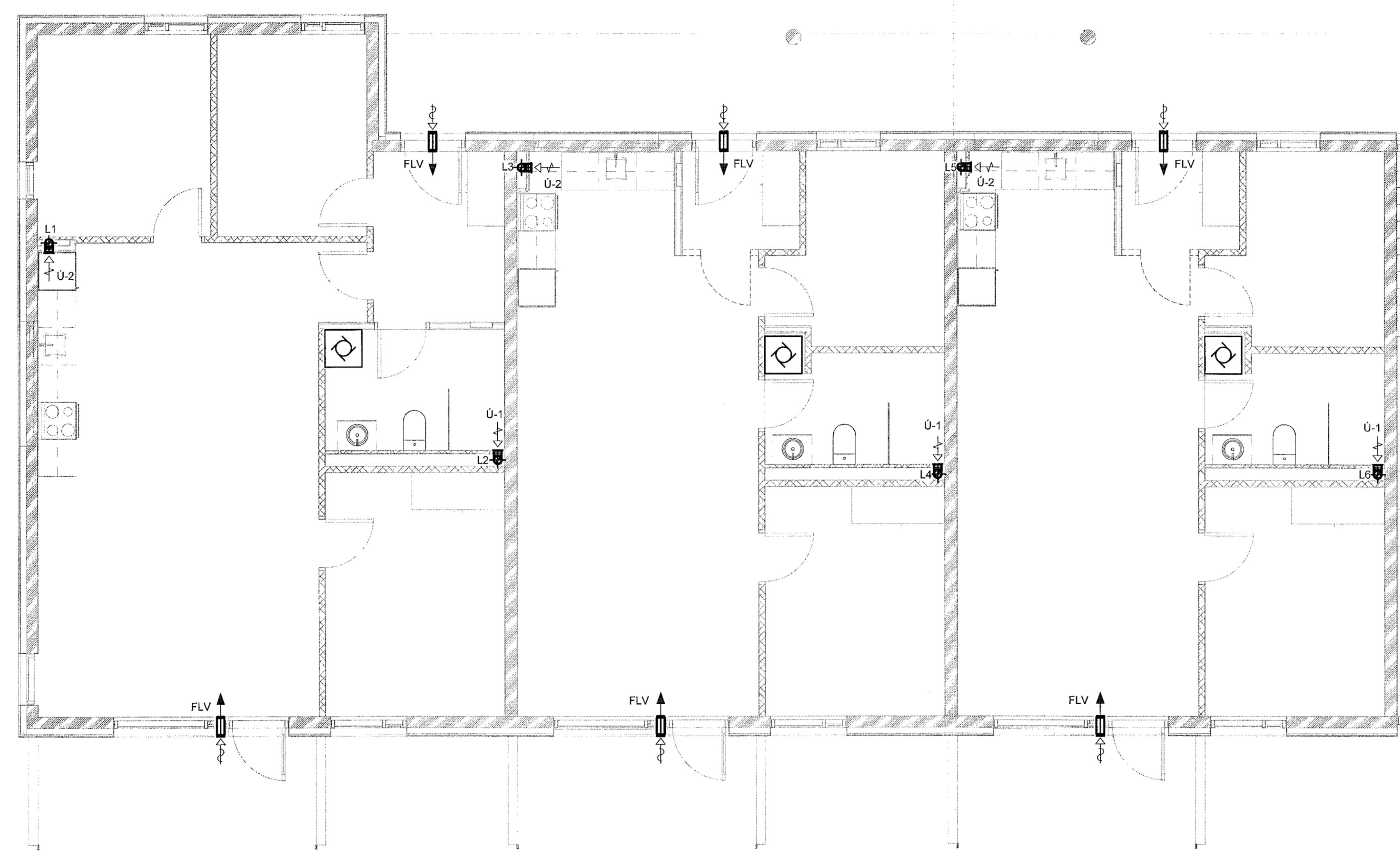
1 1.Hæð - 1 1 : 50
