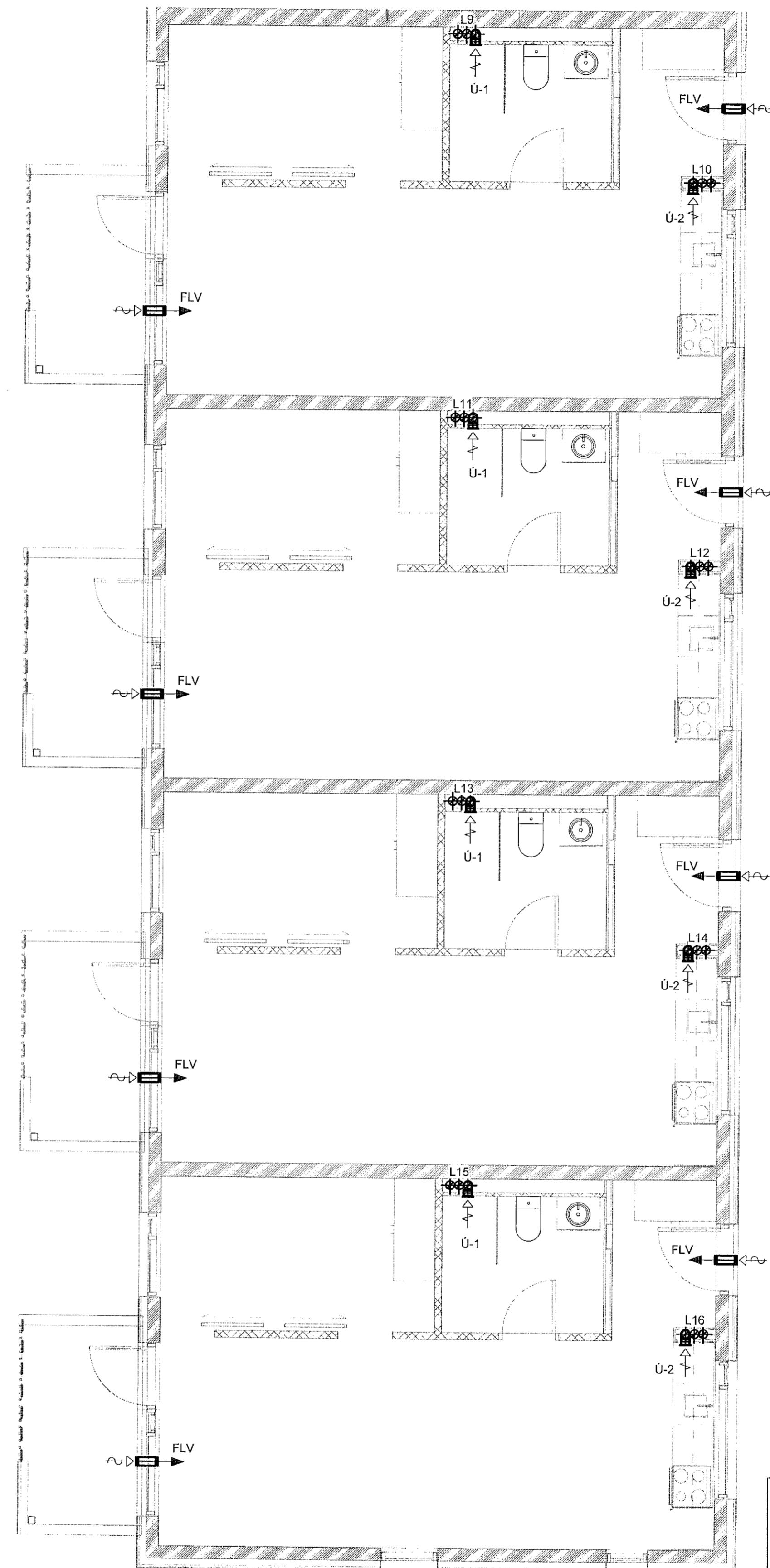
2 3. hæð - 3 1 : 50
