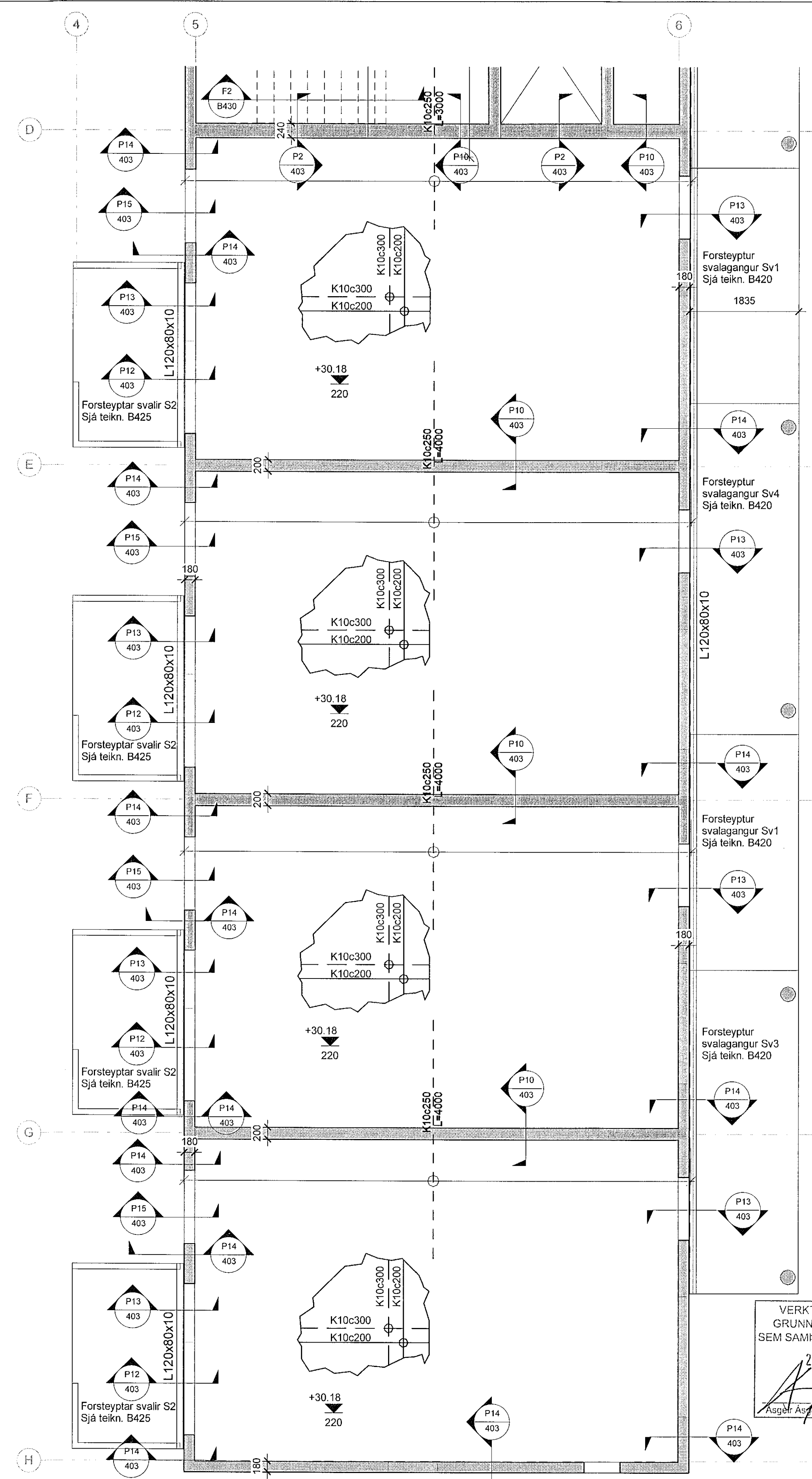
2 1.hæð - Loftaplata og veggir - 3/3 1 : 50
