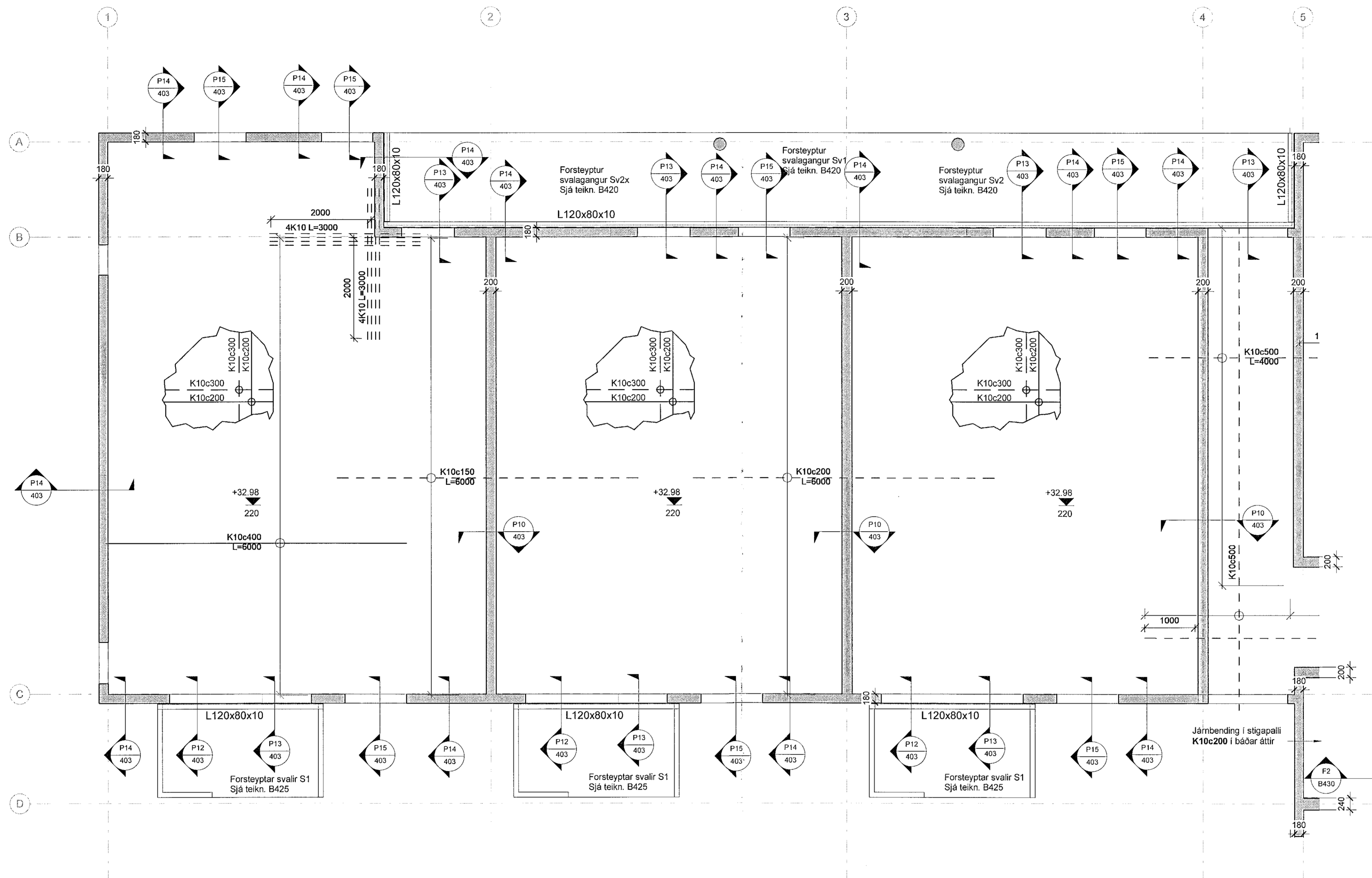
1 2.hæð - Loftaplata og veggir - 1/3 1: 50
