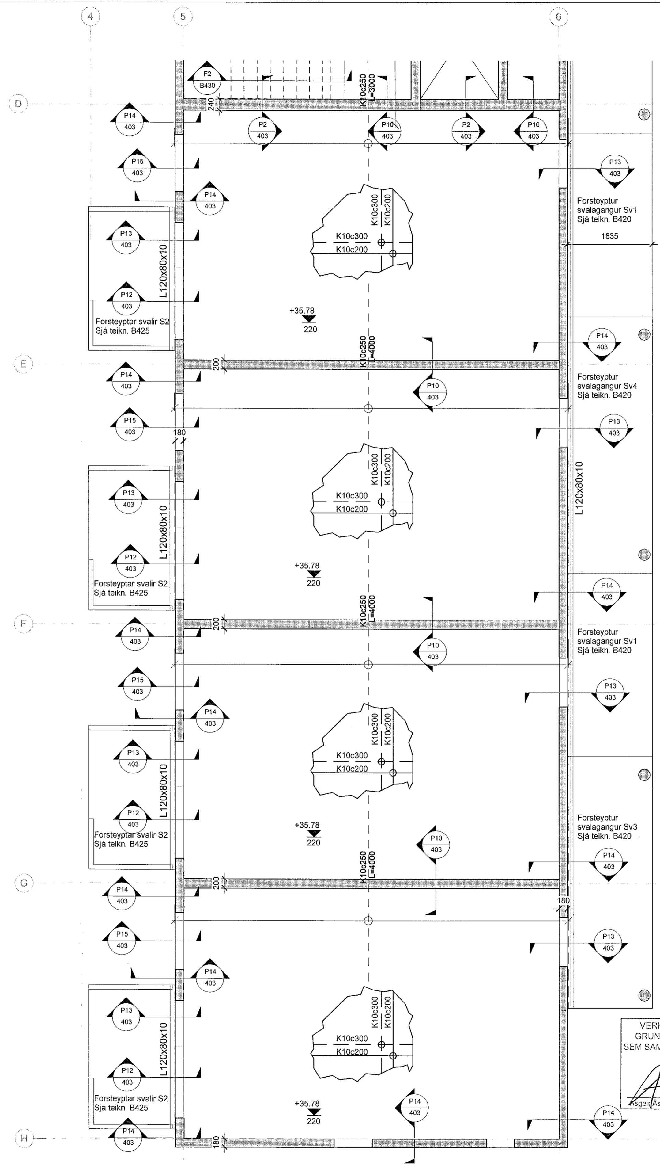
2 3.hæð - Loftaplata og veggir - 3/3 1 : 50
