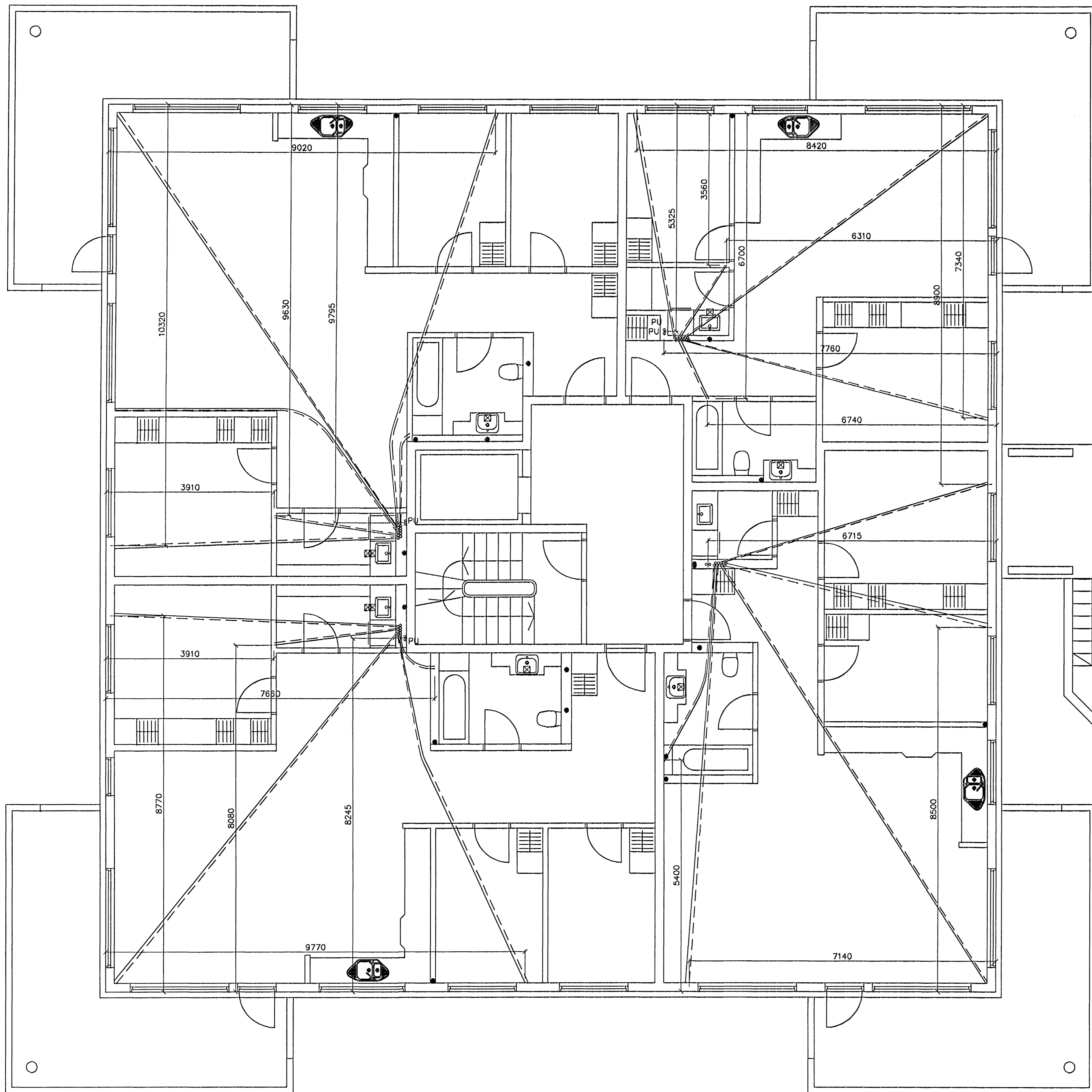
GRUNNMYND 2 HÆÐAR 1:50
