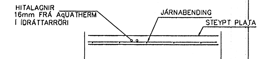
LAGNIR, SNIÐ, 1:20
