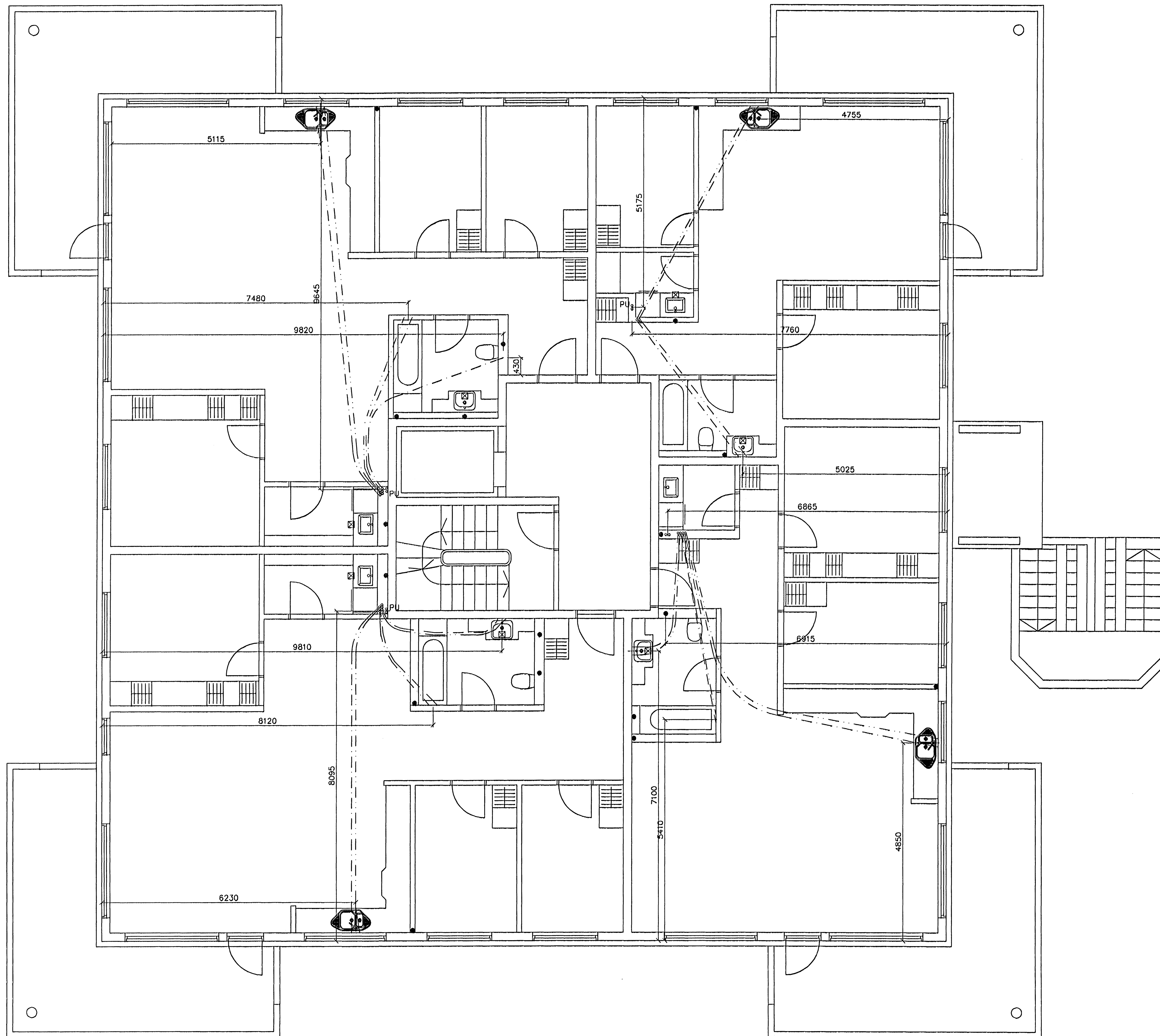
GRUNNMYND 2 HÆÐAR 1:50
