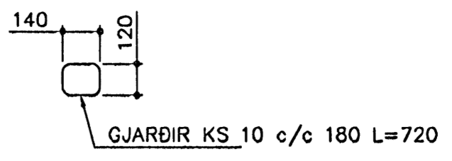
SÚLA S2 1:20
