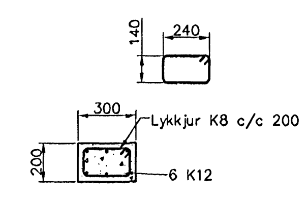
Síla S.1 1:20 1-06
