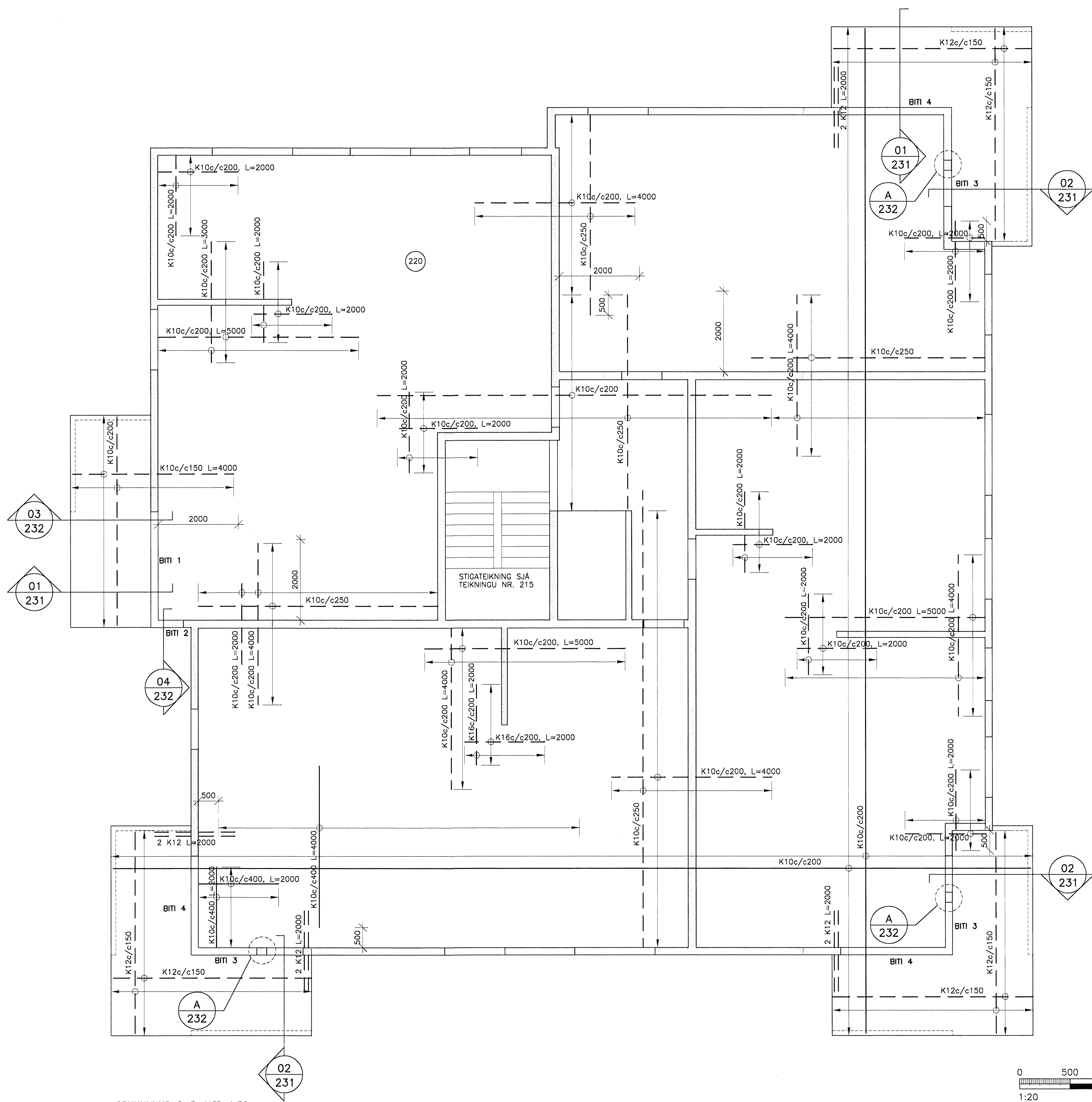
GRUNNMYND 2-5. HÆÐ 1:50
