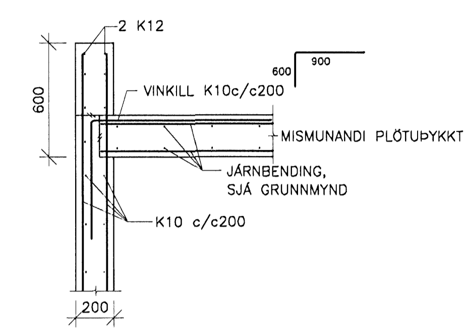
01 SNID 261 1:20
