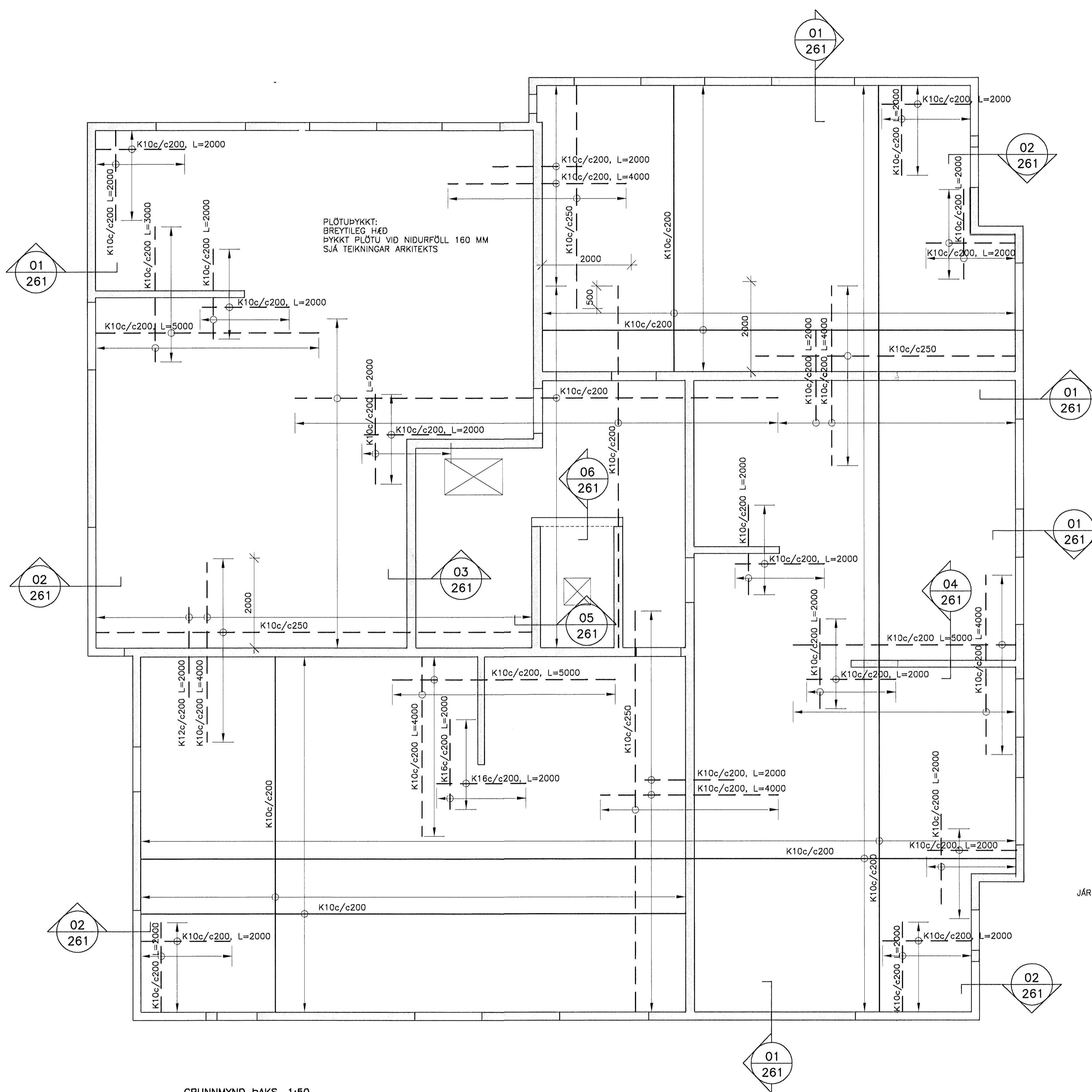
GRUNNMYND ÞAKS, 1:50
