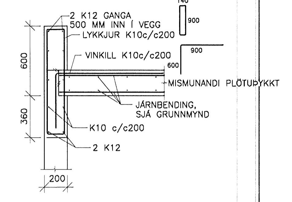
02 SNID 261 1:20
