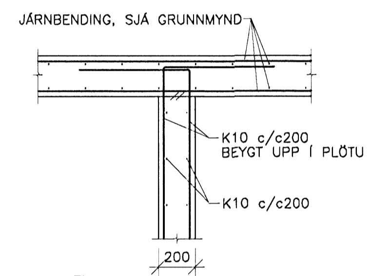
03 SNID 261 1:20
