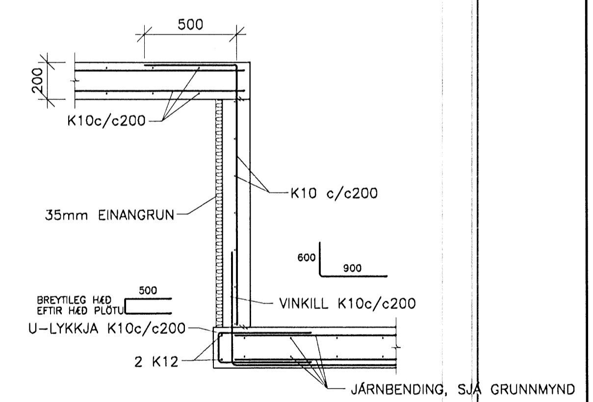
06 SNID 261 1:20
