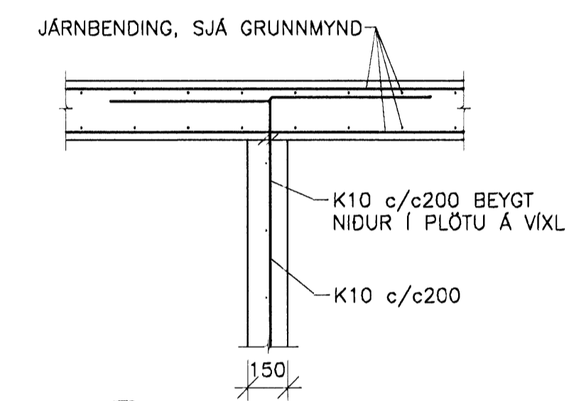
04 SNID 261 1:20
