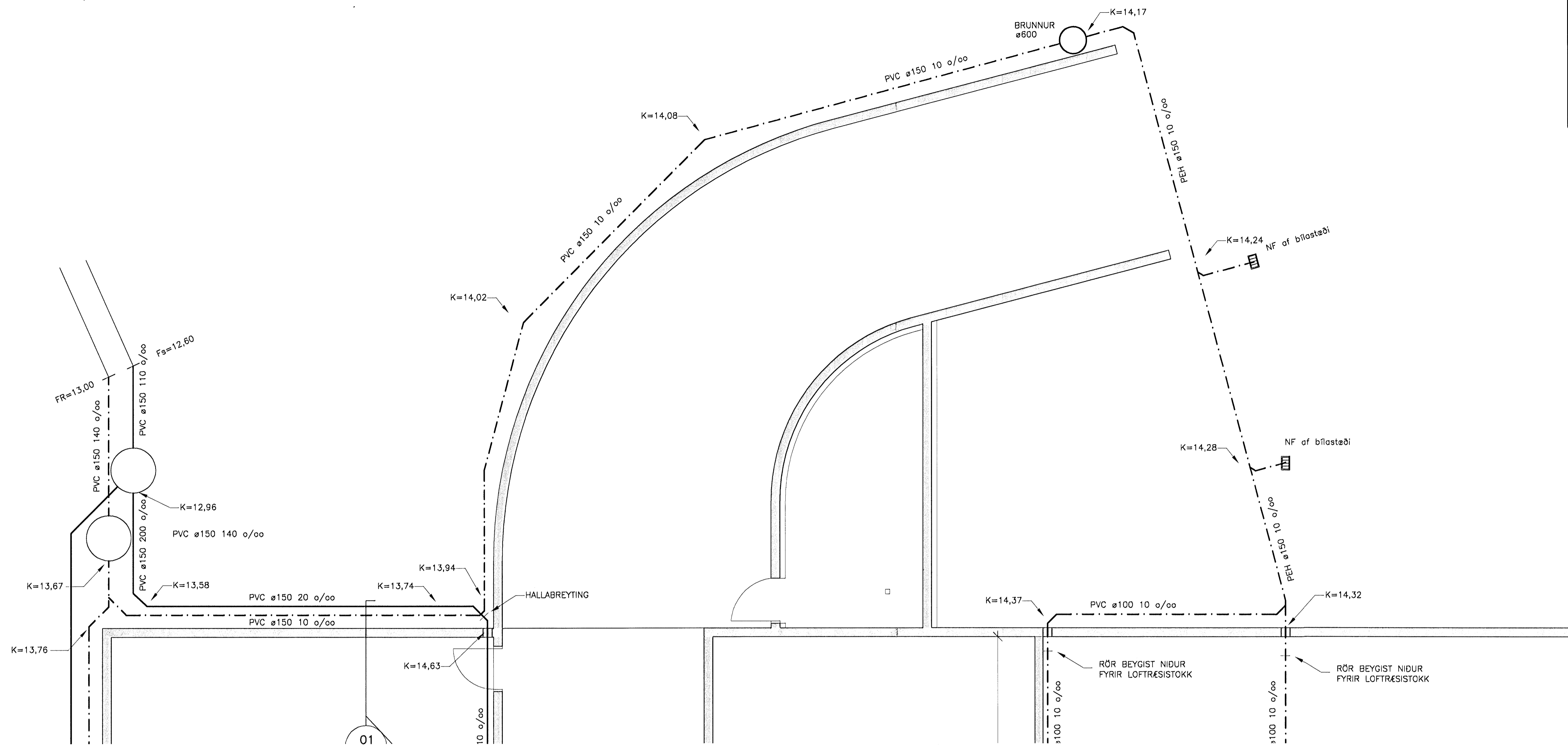
GRUNNMYND KJALLARA, 1:50
