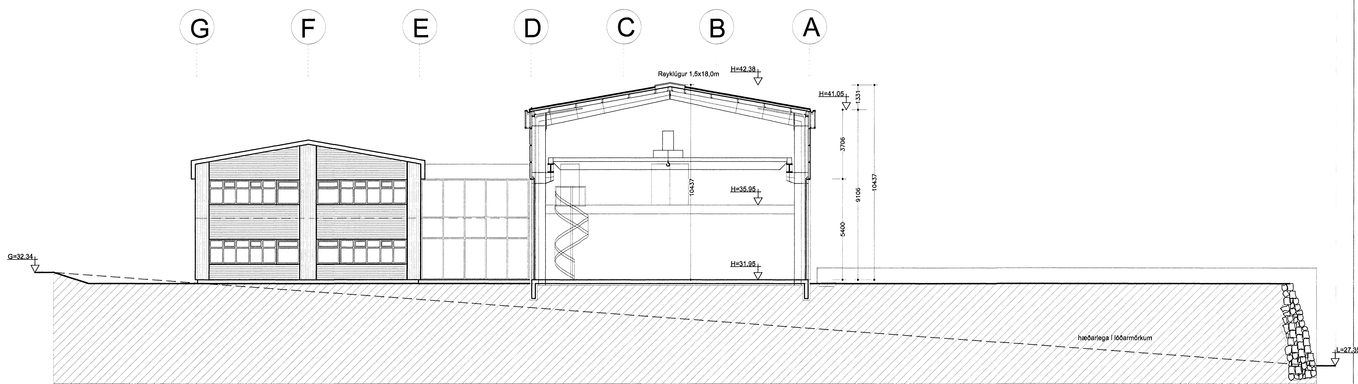
snið A-A
