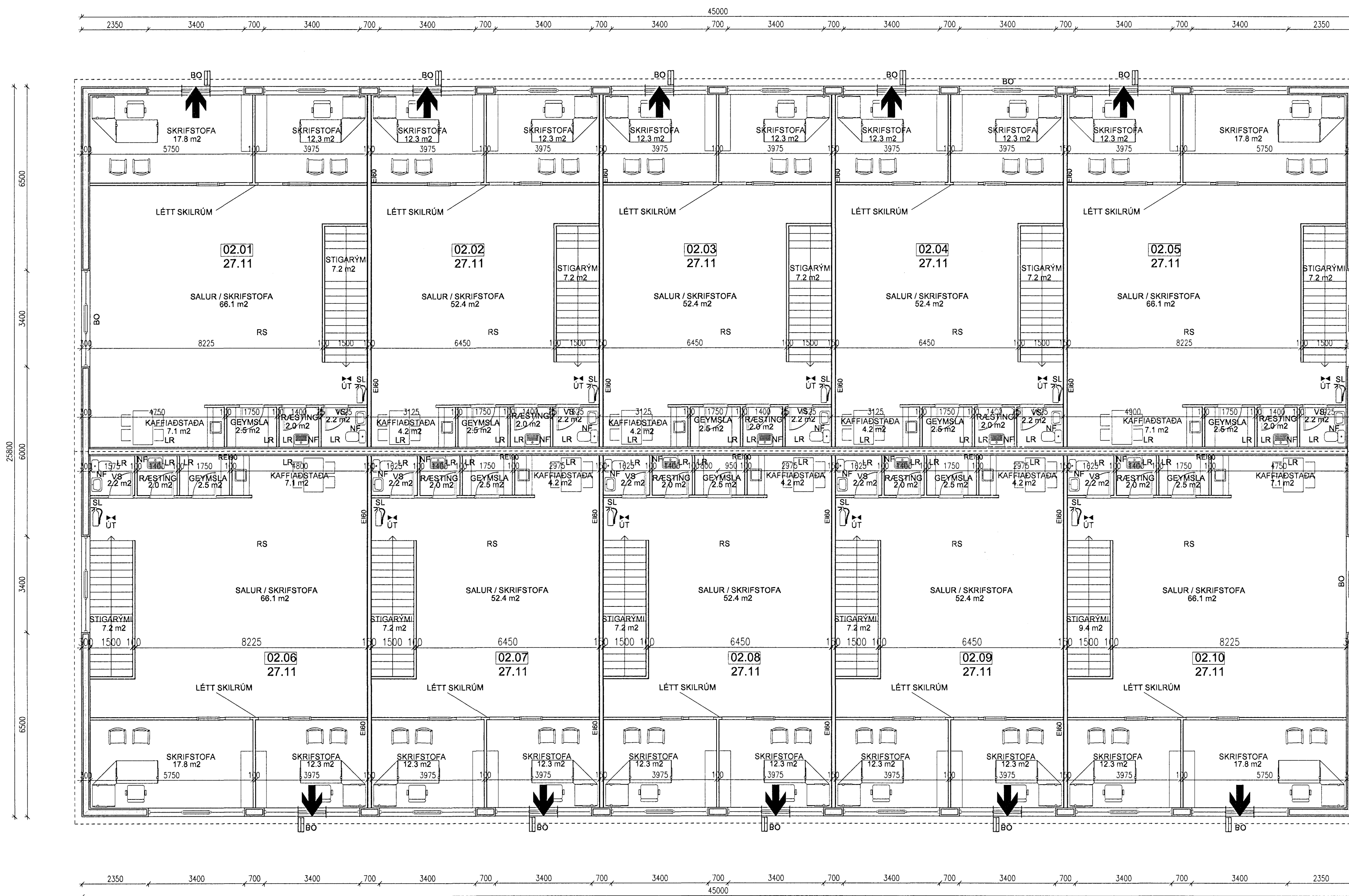
GRUNNMYND 2. HÆÐ
