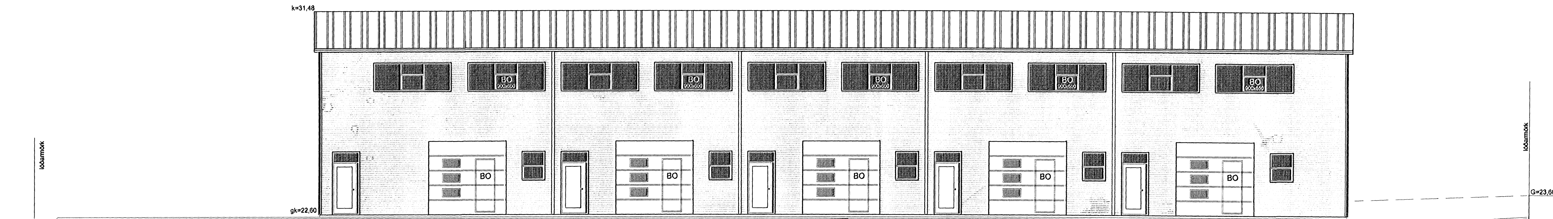
ÚTLIT VESTUR 1:100 L=20,00 G=22,05
