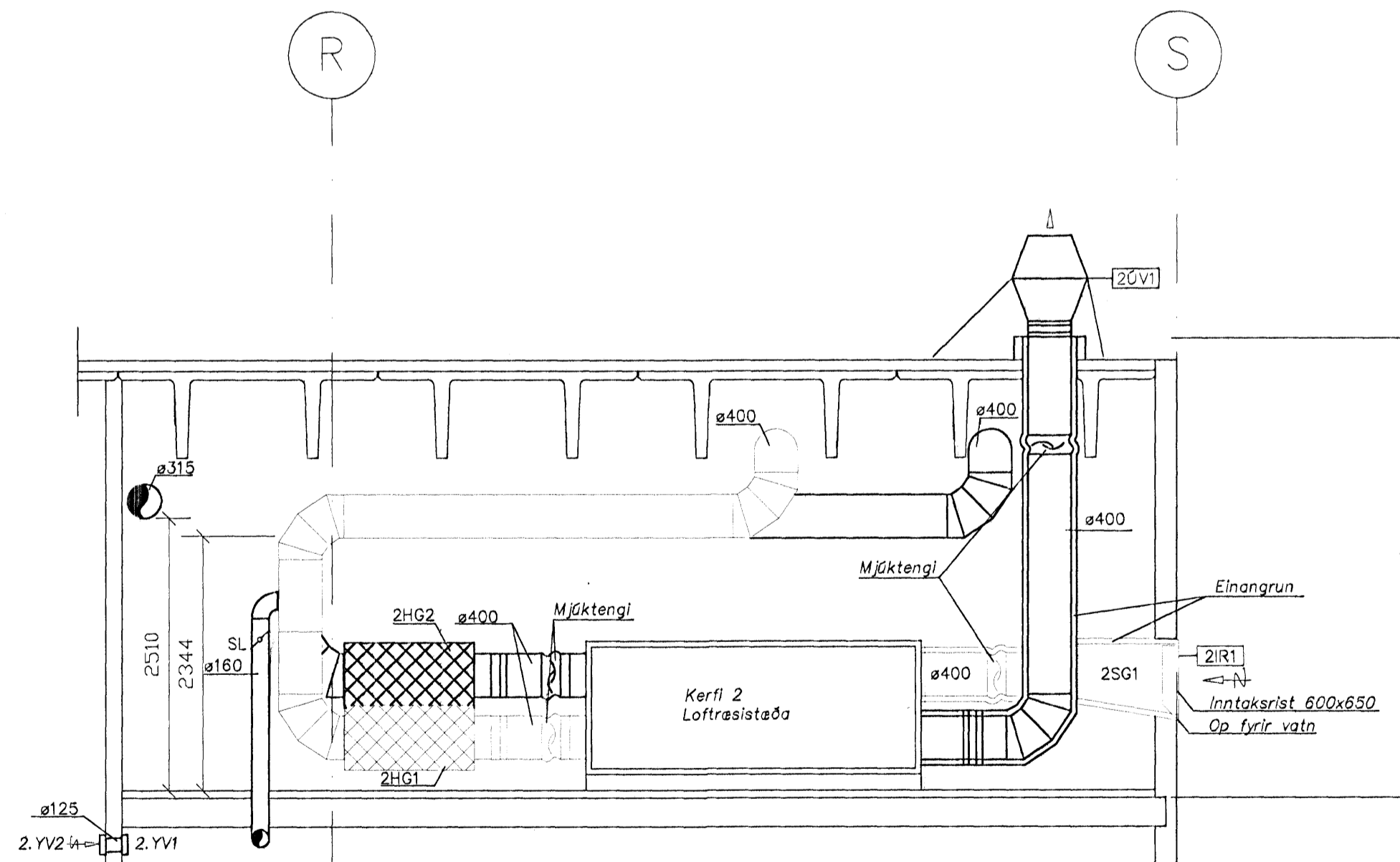
Snið C-C
