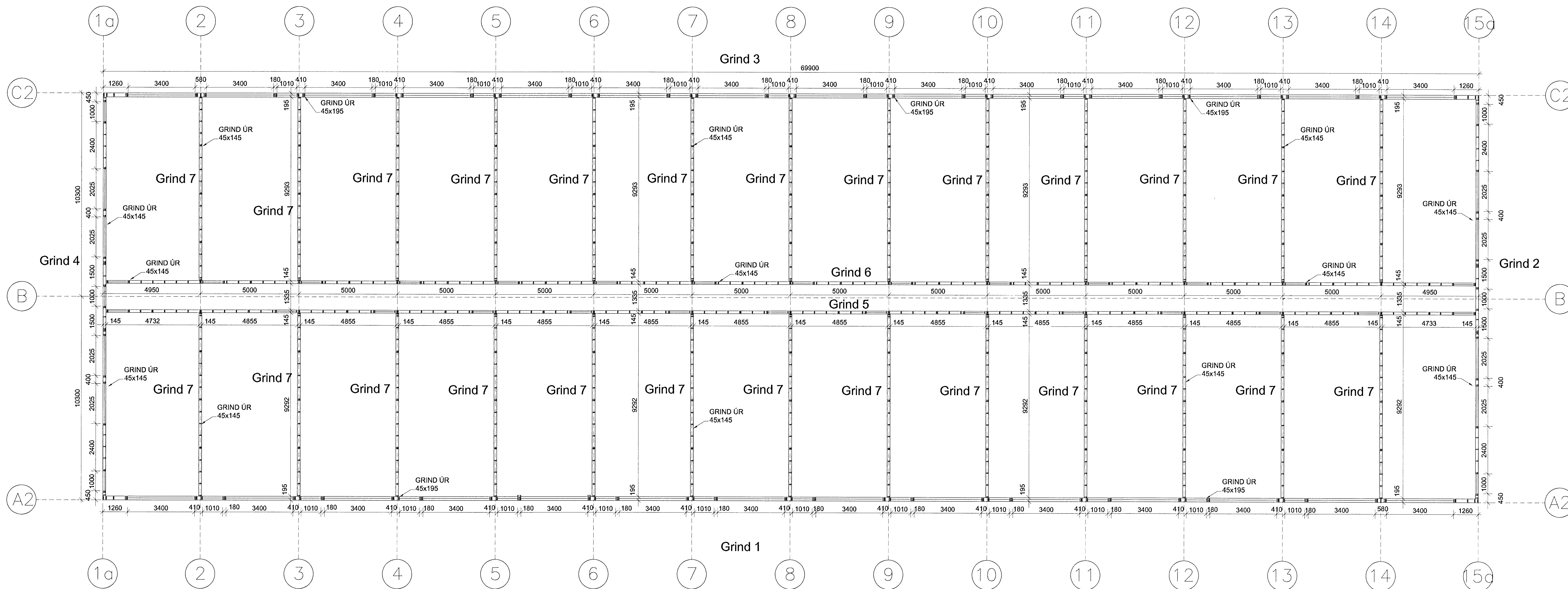
GRUNNMYND NEDRI HÆÐ 1:100
