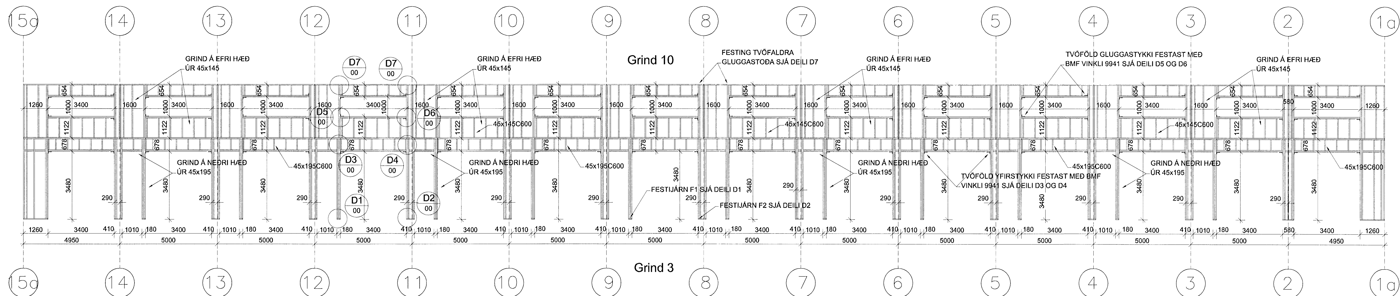
ÚTVEGGUR BAKHLÍÐ 1:100 GRIND 3 OG 10
