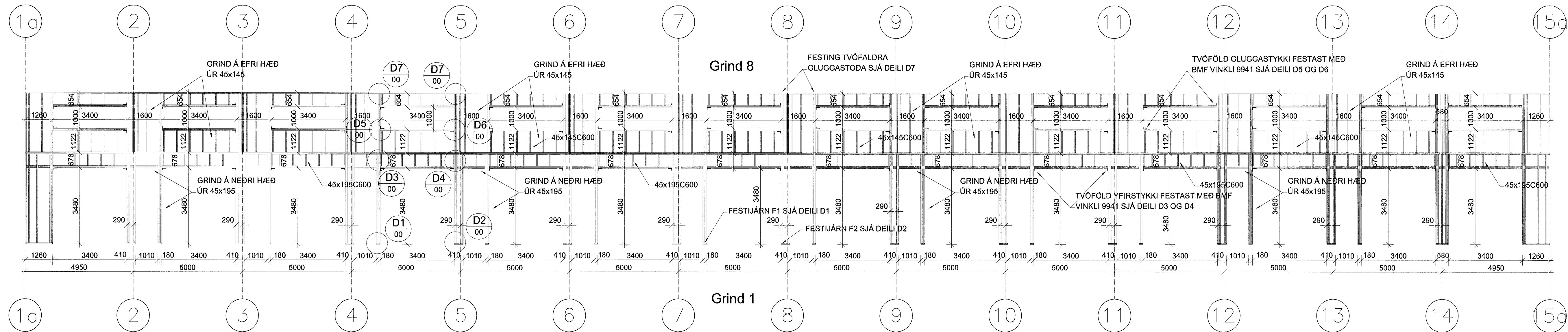
ÚTVEGGUR FRAMHLÍÐ 1:100 GRIND 1 OG 8
