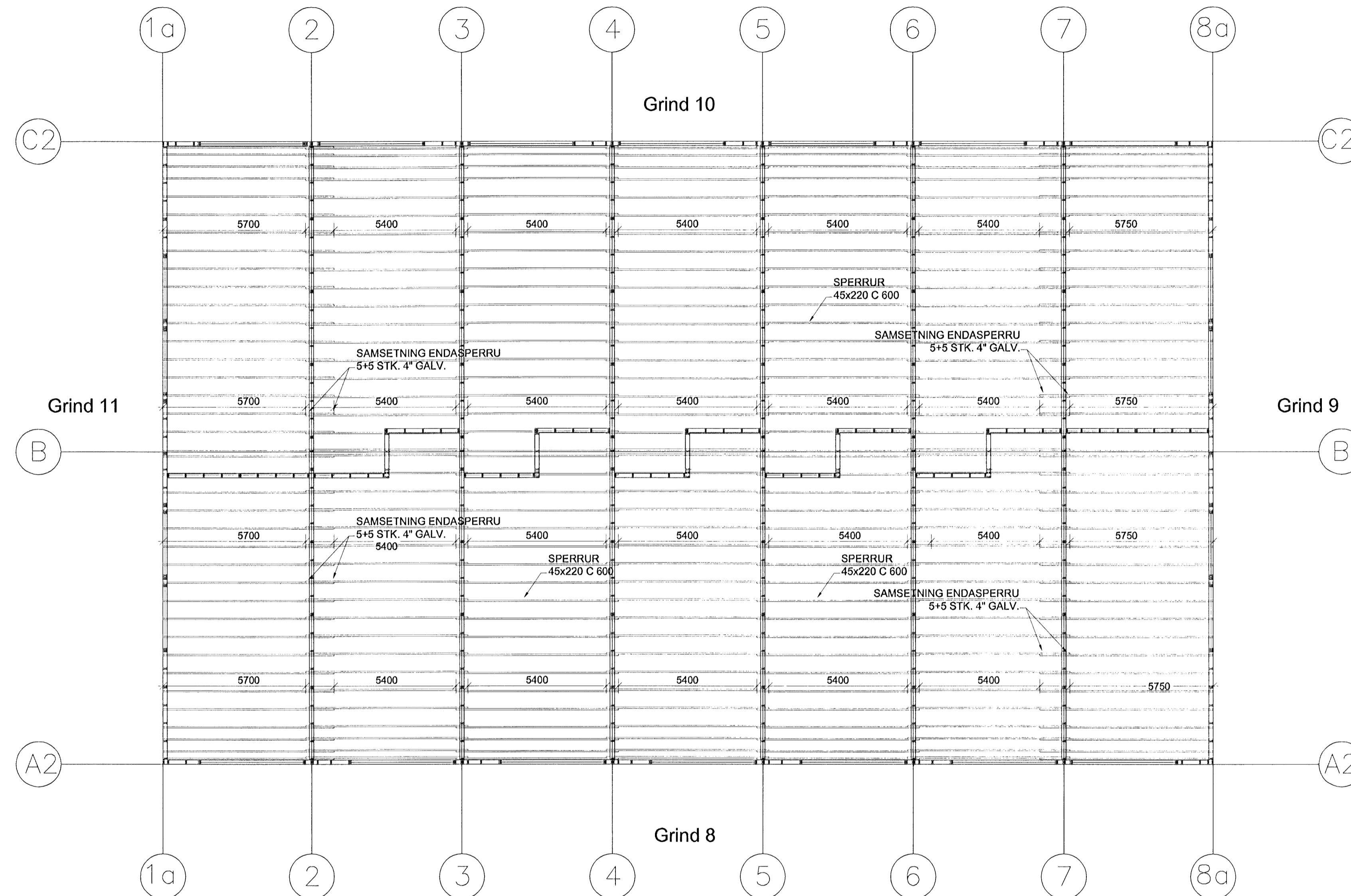
ÞAKSPERRUR GRUNNMYND 1:100
