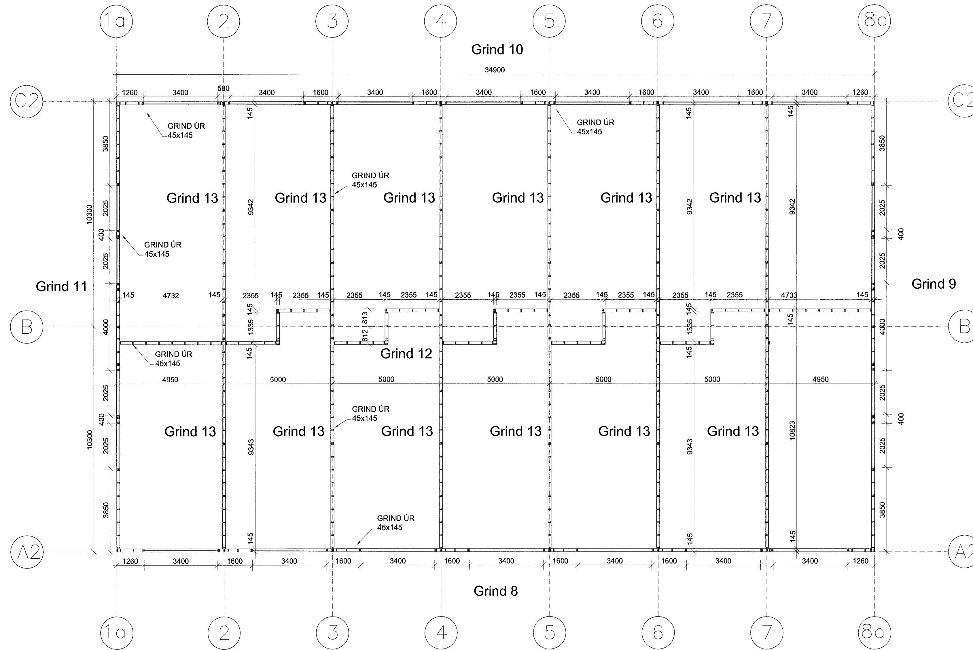
GRUNNMYND EFRI HÆÐ 1:100
