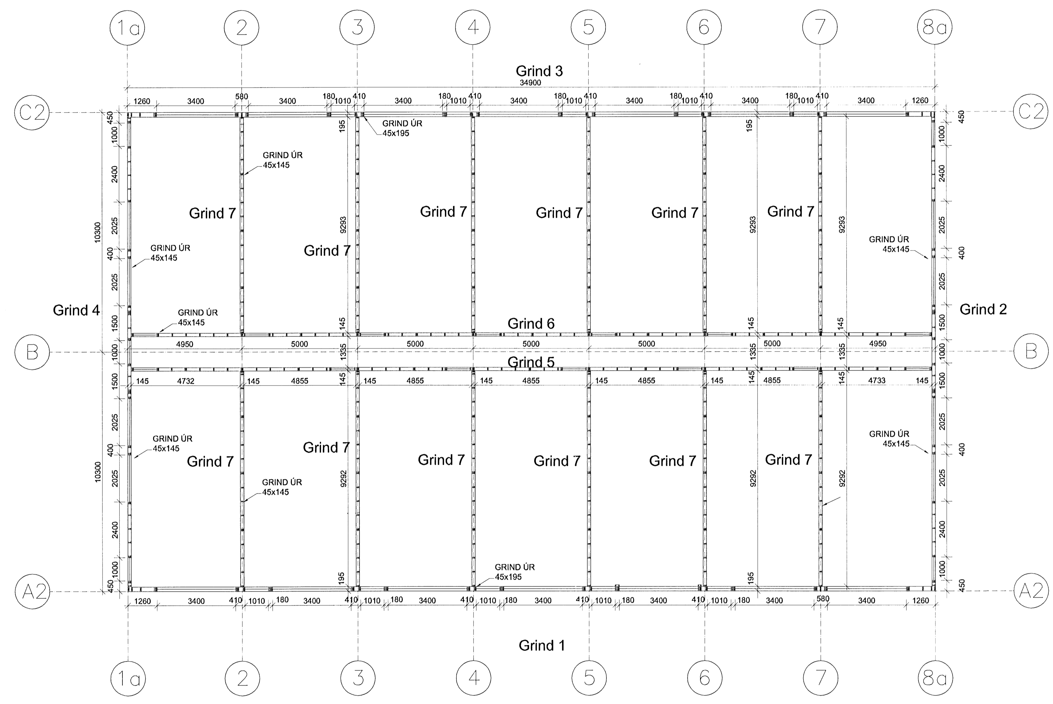
GRUNNMYND NEDRI HÆÐ 1:100
