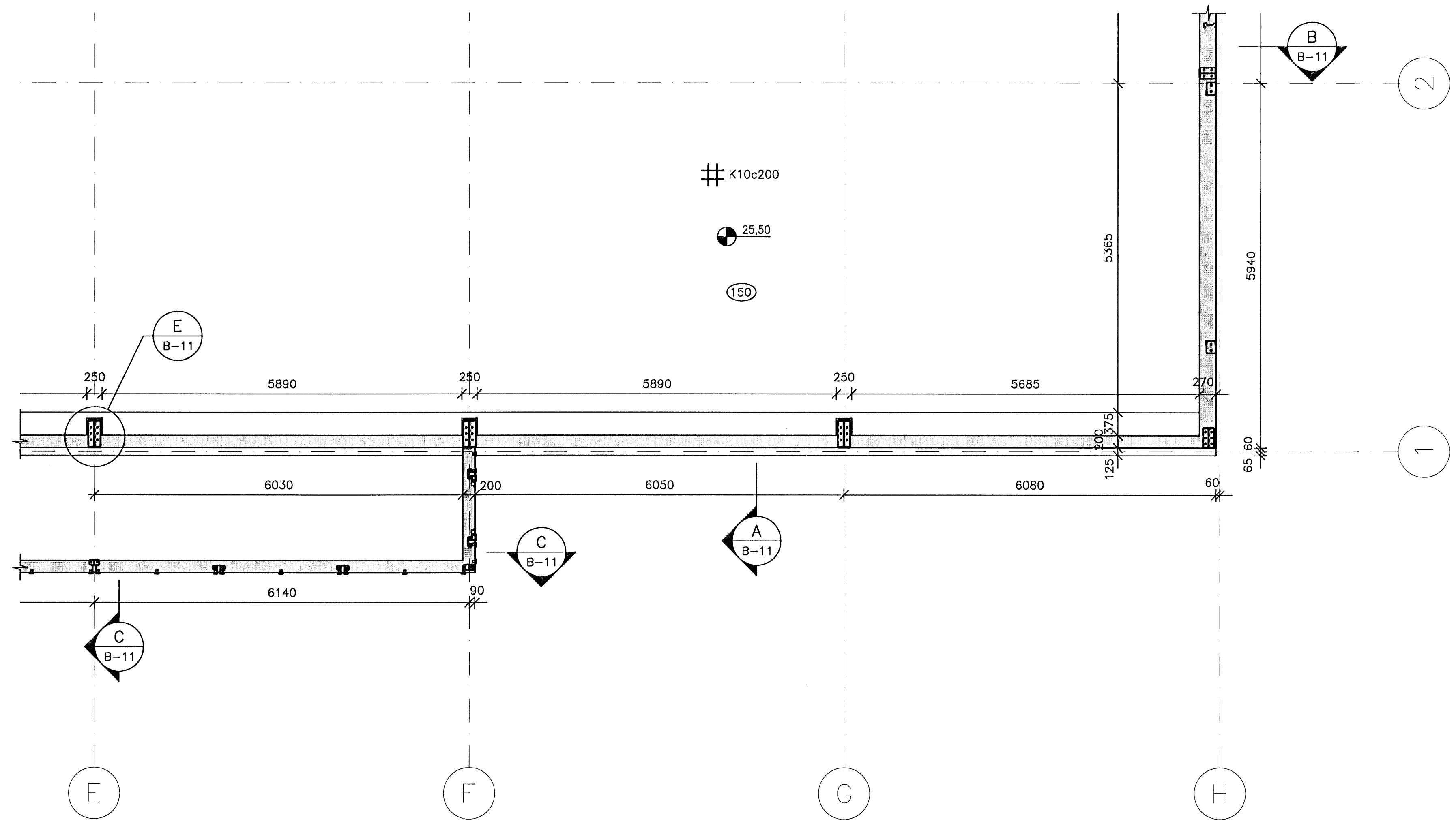
GR Grunnmynd 4 - 1:50
