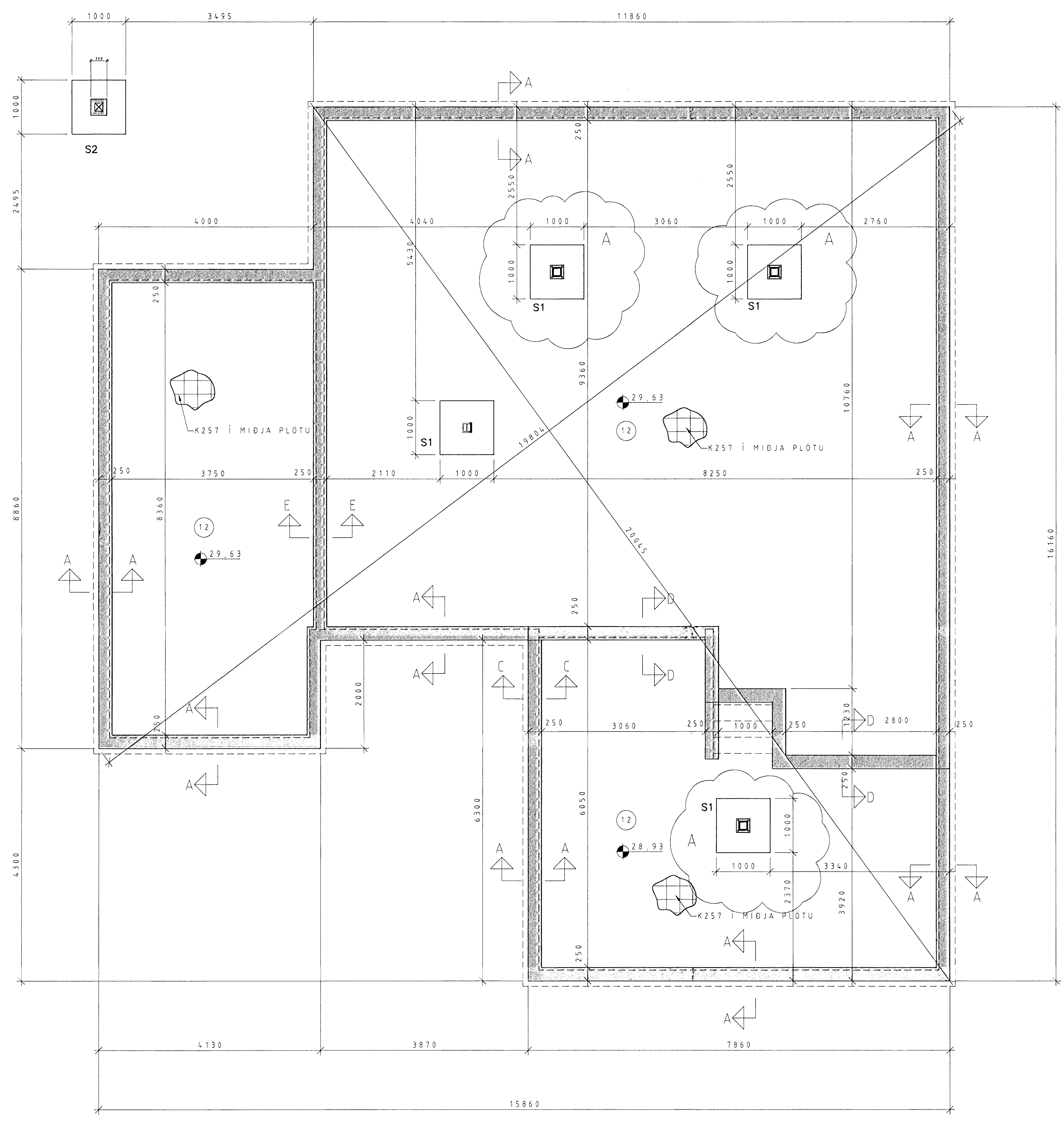
GRUNNMYND SÖKKLA 1 :50
