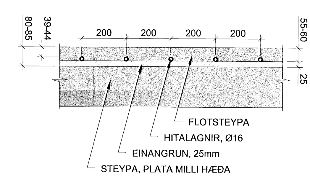
SM2 GÓLFHITALAGNIR 2. HÆÐ 1:10 DÆMIGERT ÞVERSNIÐ
