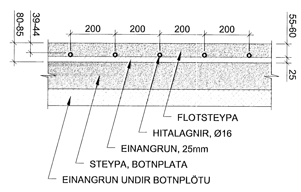
GÓLFHITALAGNIR, DREIFIKISTA 2
