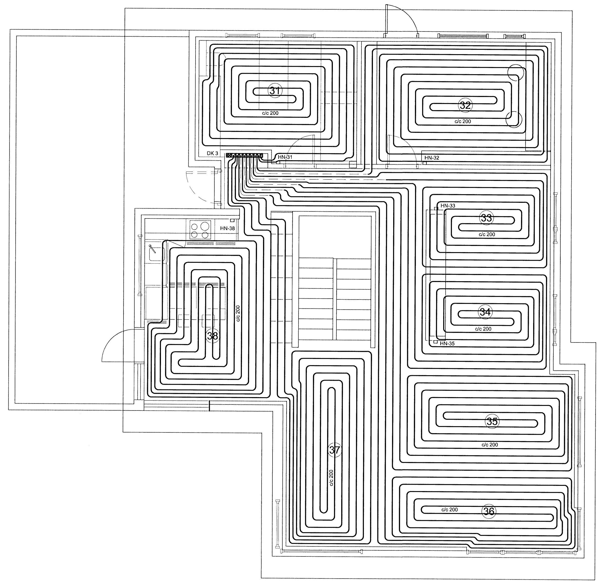
GRUNNMYND - 2. HÆÐ
