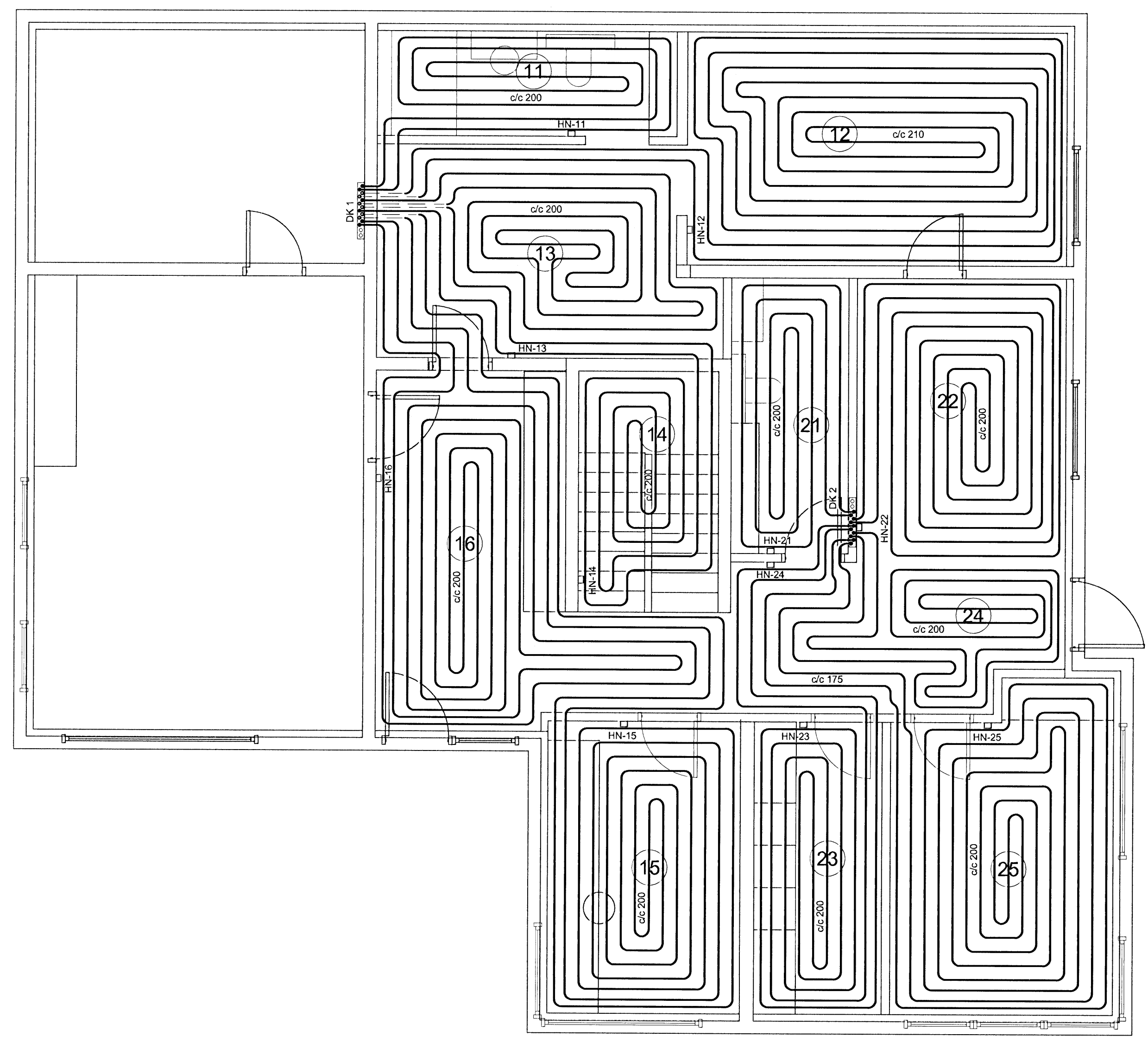
GRUNNMYND - 1. HÆÐ
