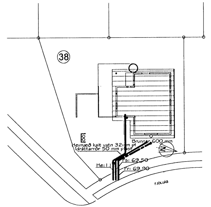
Afstöðumynd 1: 500
