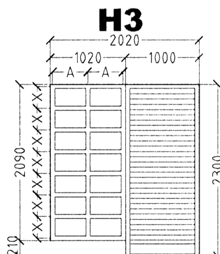
1. STK. ANDDYRI. HURÐ OPNAST VINSTRI INN.
